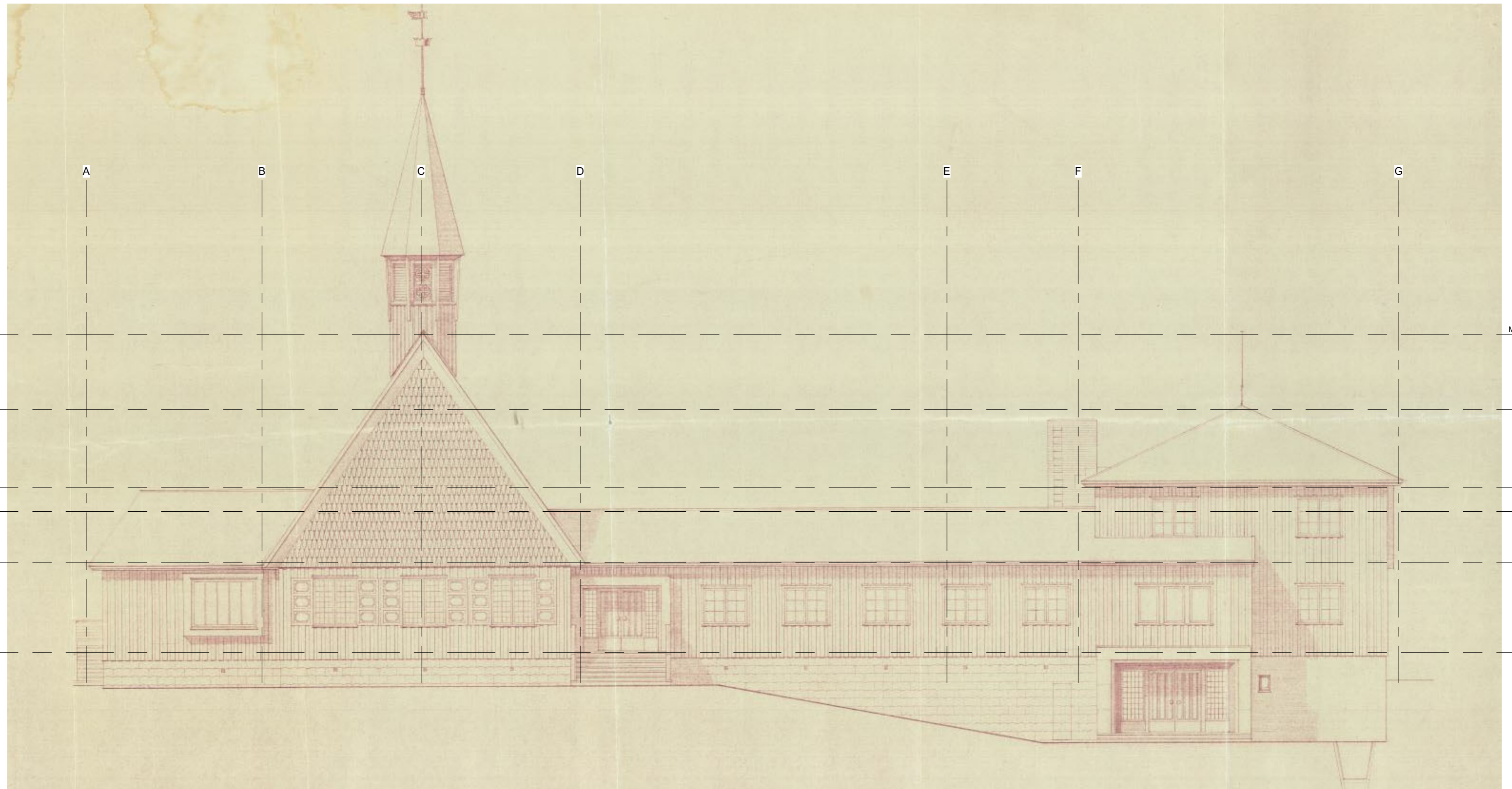
A40_03 - Fasade Øst 1 : 100
