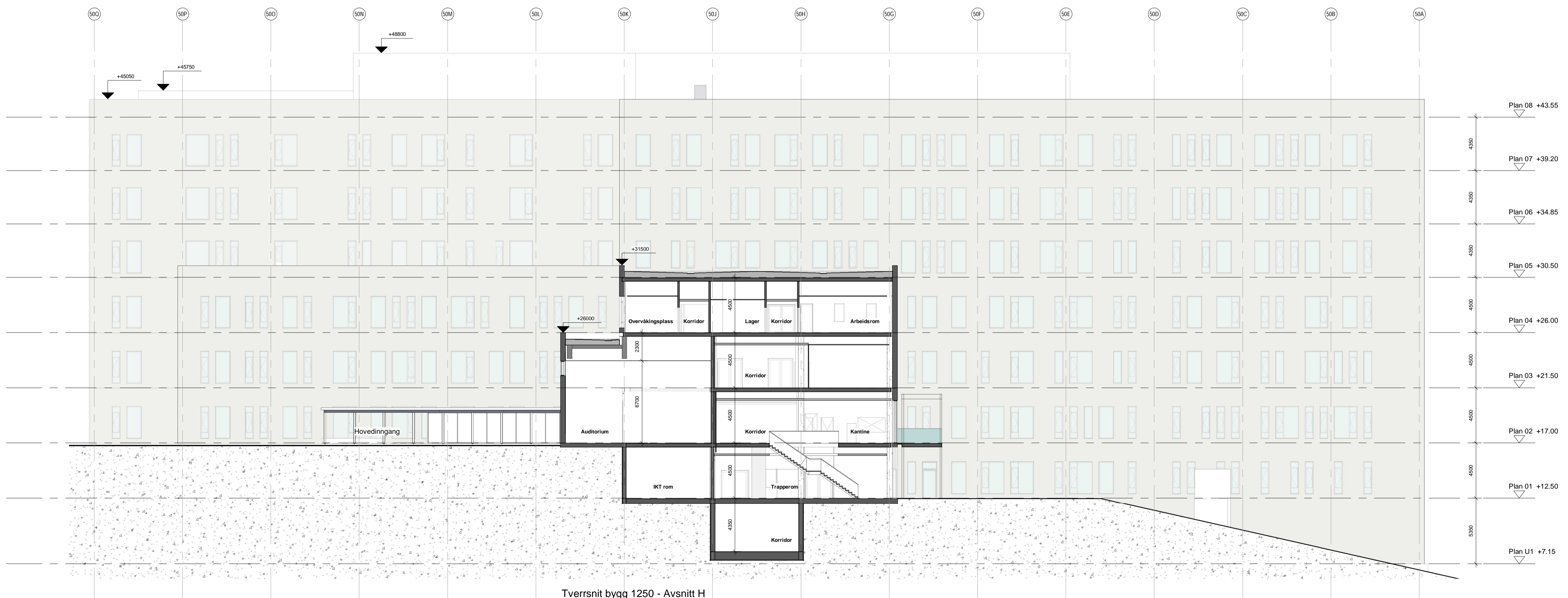
Tversnitt bygg 1250 - Avsnitt H
