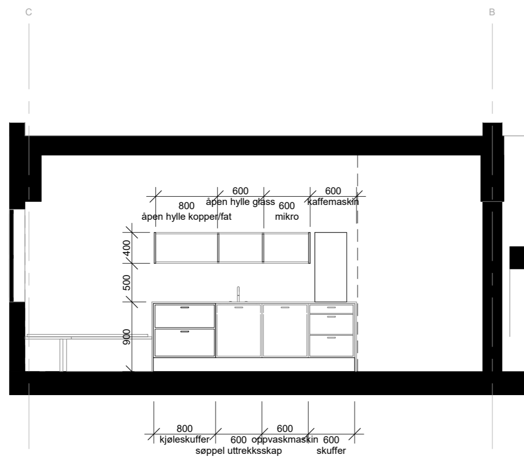
Oppriss kjøkken 1 : 50
