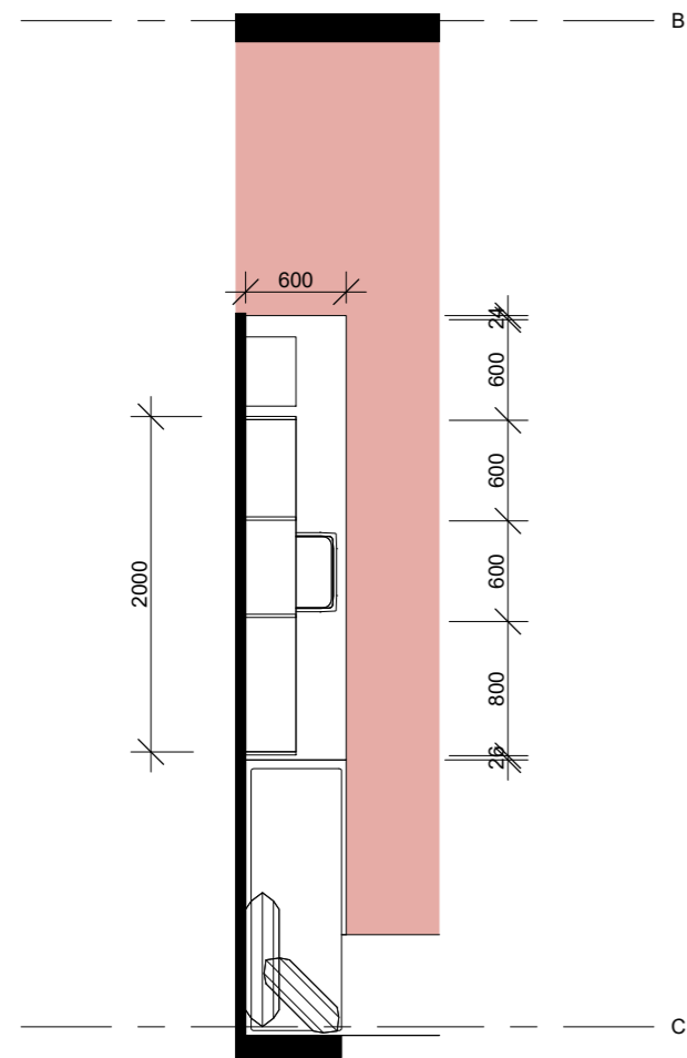
Utsnitt 1 1 : 50
