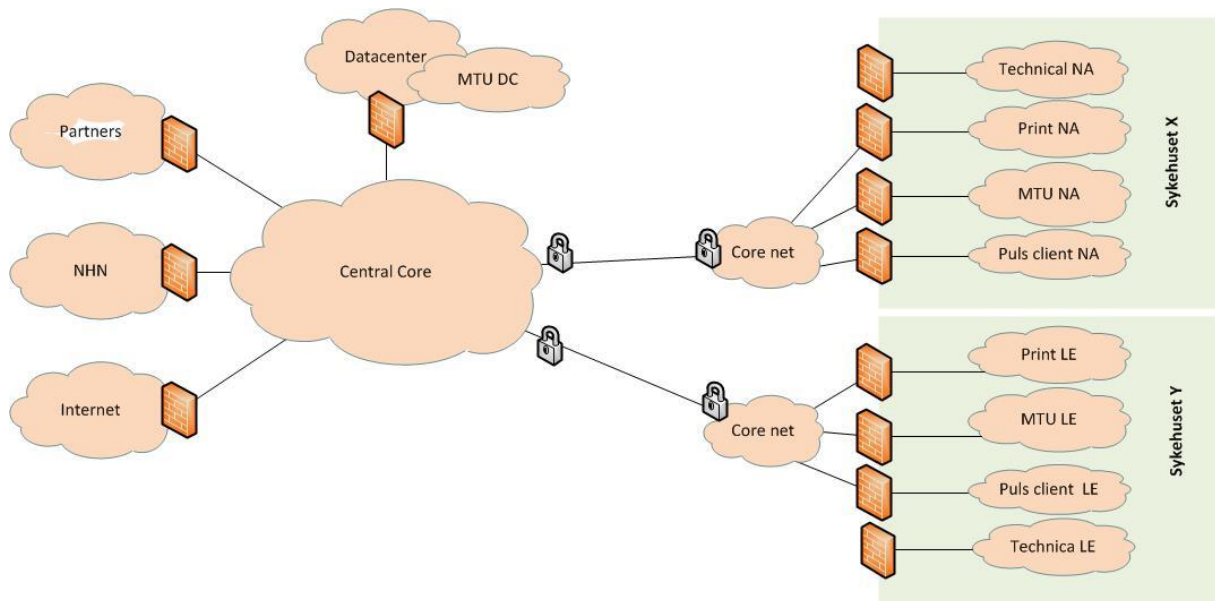
Figur 1 - Virtual LAN
