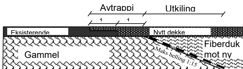
Figur 7.10 Utkiling ved endeavslutning
