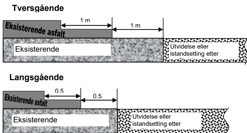
Figur 11.3 Avtrapping mot eksisterende asfalt før asfaltering ved henholdsvis tversgående og langsgående skjøter
