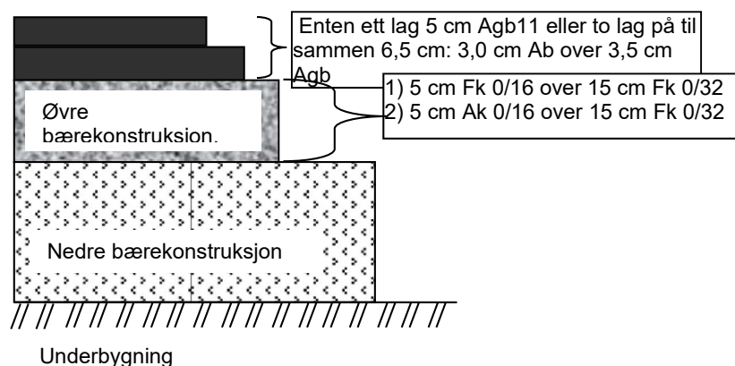
Figur 7.4 Alternative oppbygninger for skulder
