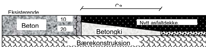
Figur 7.12 Utkiling ved overgang mellom asfalt og betong
