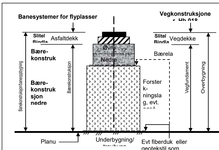
Figur 6.1 Prinsippsskisse som angir de mest vanlige benyttede begrep og materiallag i bærekonstruksjonen
