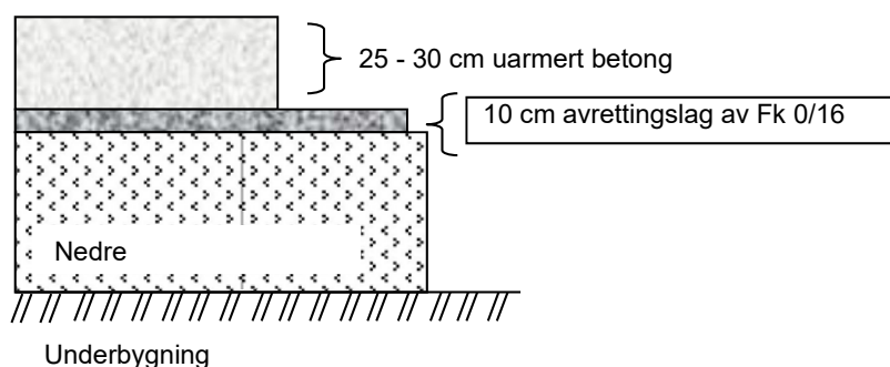
Figur 7.6 Alternative oppbygninger av betong for store flyplasser
