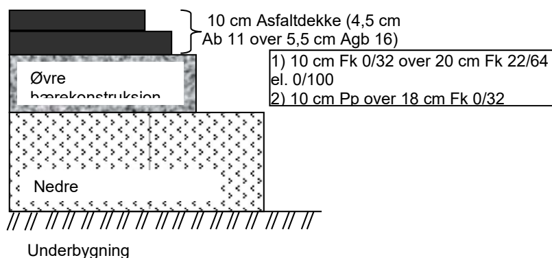
Figur 7.3 Alternative oppbygninger ved forlengelse av rullebane for ringtrykk mellom 1,0 og 1,5 MPa
