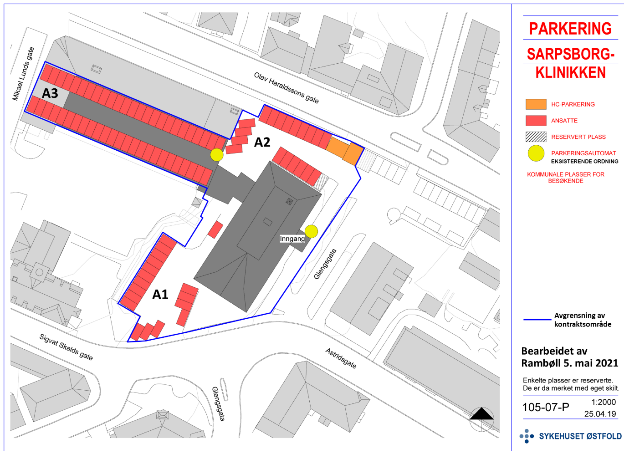
Figur 7 Kontraktssområde og disponering av parkeringsområder ved Sykehuset Østfold Sarpsborgklinikken (Grunnlag tegn. 105-07-P av 24.04.2019)
