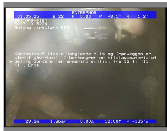
Foto: 5820_5224_5227_05022021_064429.JPG 23,27m, Korrosjon/Slitasje, Manglende tilslag (rørveggen er sterkt påvirket), I bertongrør er tilslagsmaterialet delvis borte eller armering synlig, fra 12 til 11 Kl., Ende
