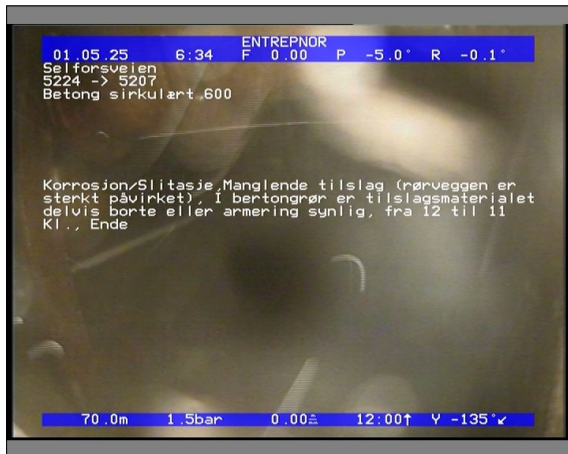
Foto: 5814_5207_5224_05022021_065637.JPG 70,02m, Korrosjon/Slitasje, Manglende tilslag (rørveggen er sterkt påvirket), I bertongrør er tilslagsmaterialet delvis borte eller armering synlig, fra 12 til 11 Kl., Ende
