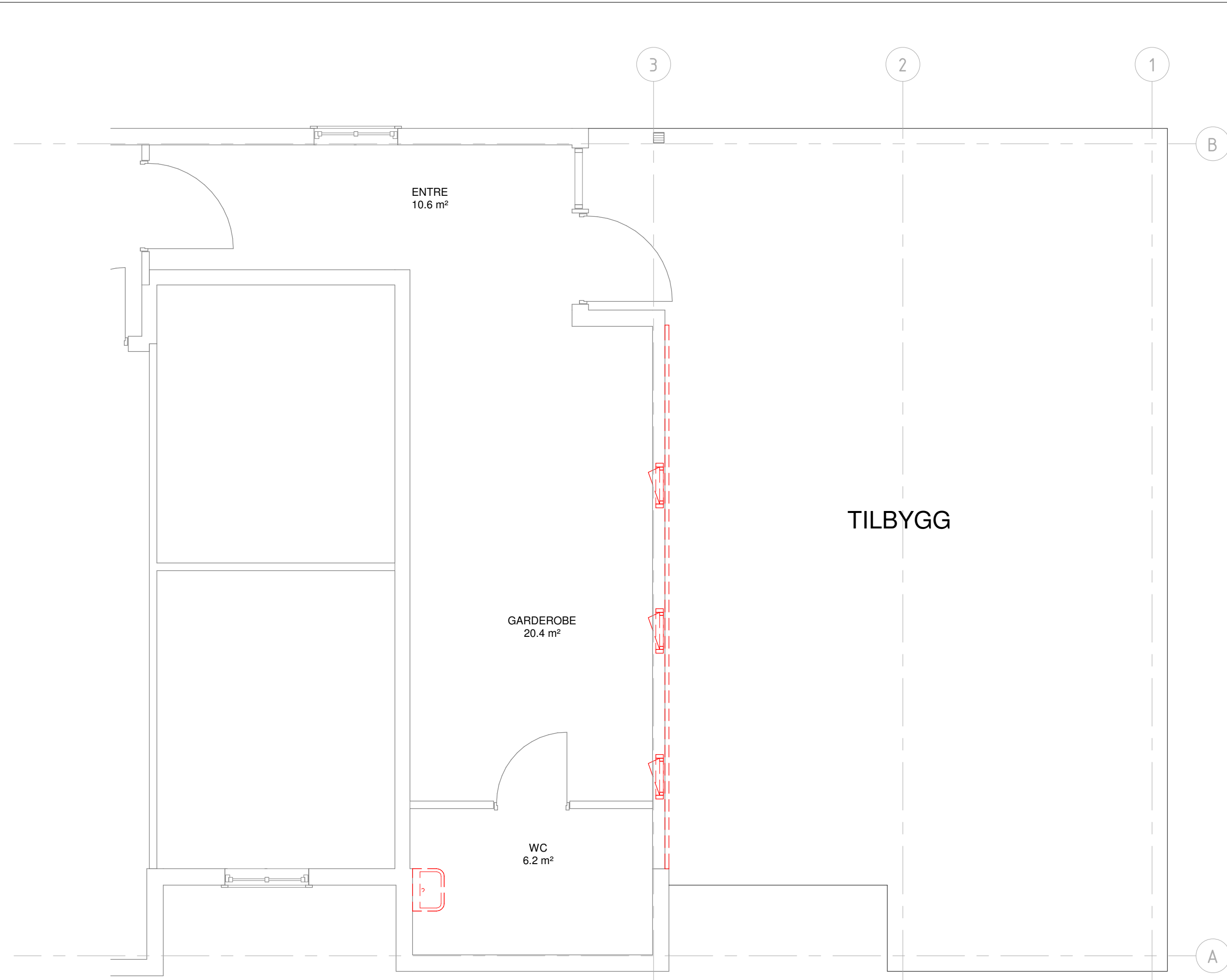
PLAN 01 RIVEPLAN 1 : 50
