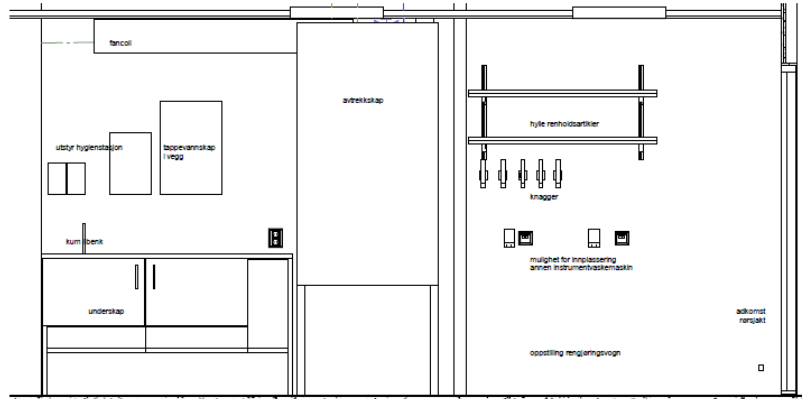
Oppriss E263 1-20 1 : 20
