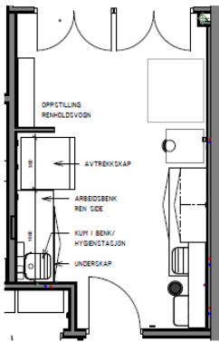
Plan E263 1 : 50
