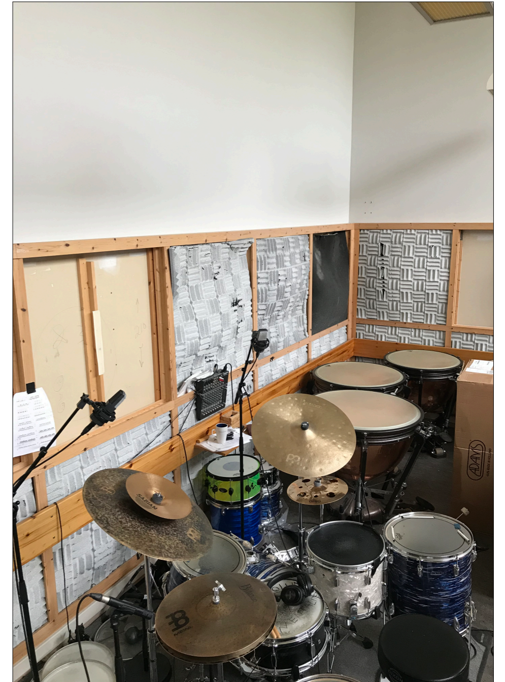
Slagverkrom - eks. veggabsorbenter med trerammer demonteres
