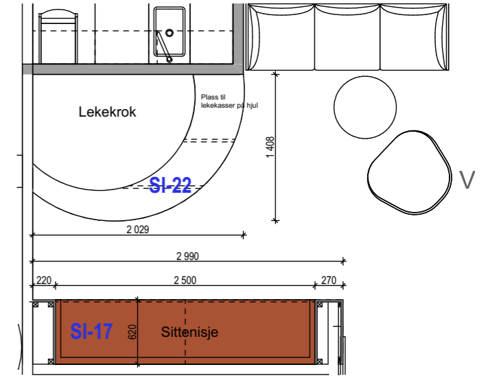
Planutsnitt:
