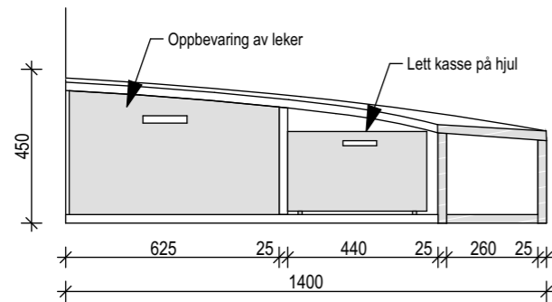
OPPRISS BB
