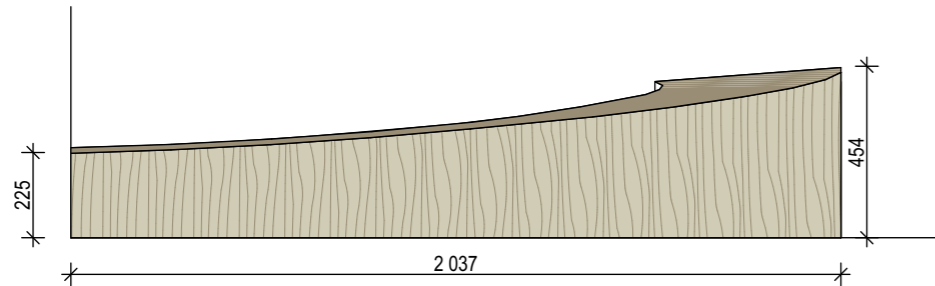
OPPRISS AA
