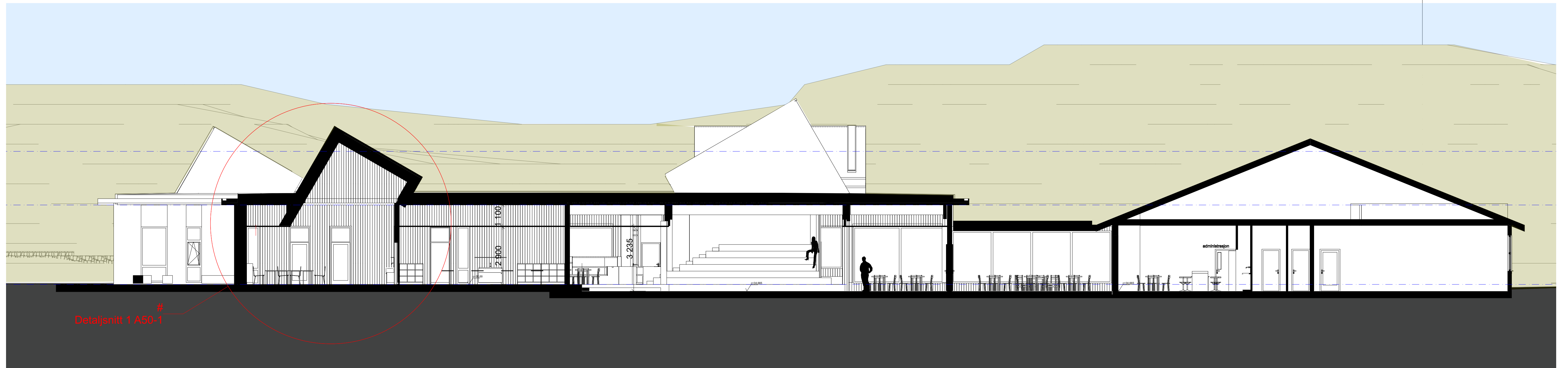
SNITT A:A
