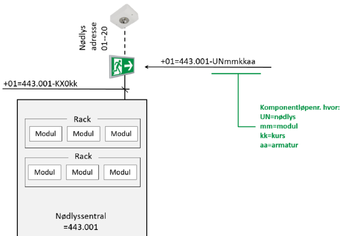
Figur 6-1 Topologiskjema for nøddlysanlegg
