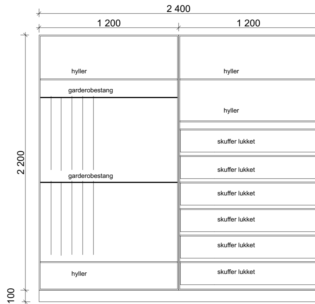
Leil 07- gard 02 1:20
