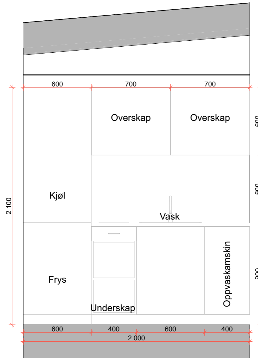
Oppriss kjøkken 1:20
