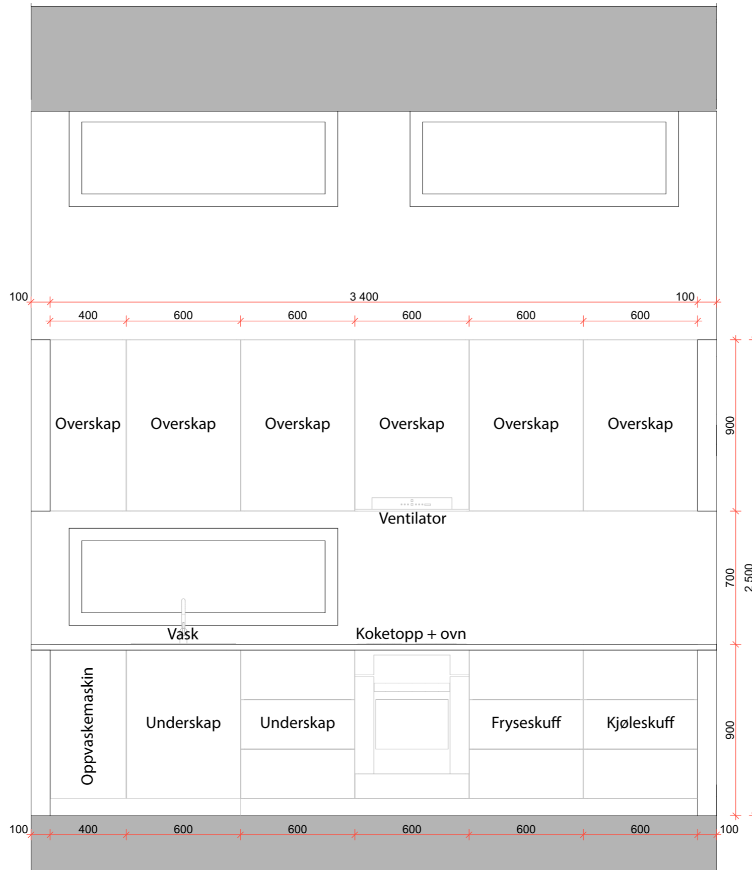
Oppriss kjøkken 1:20
