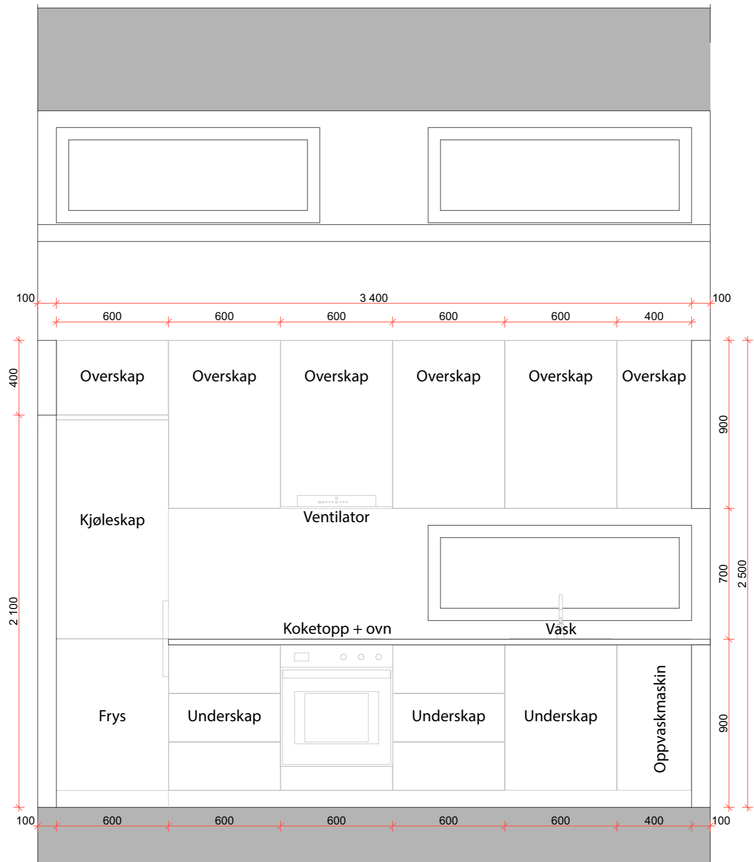
Oppriss kjøkken 1:20
