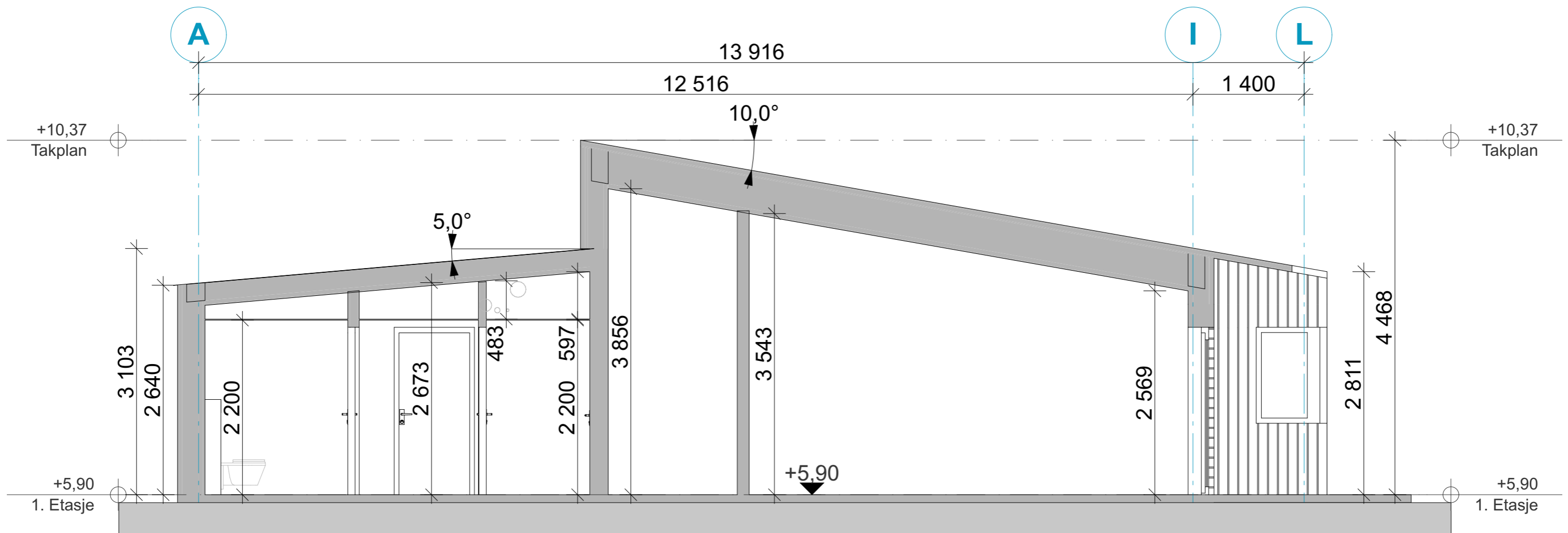
Snitt B 1:50
