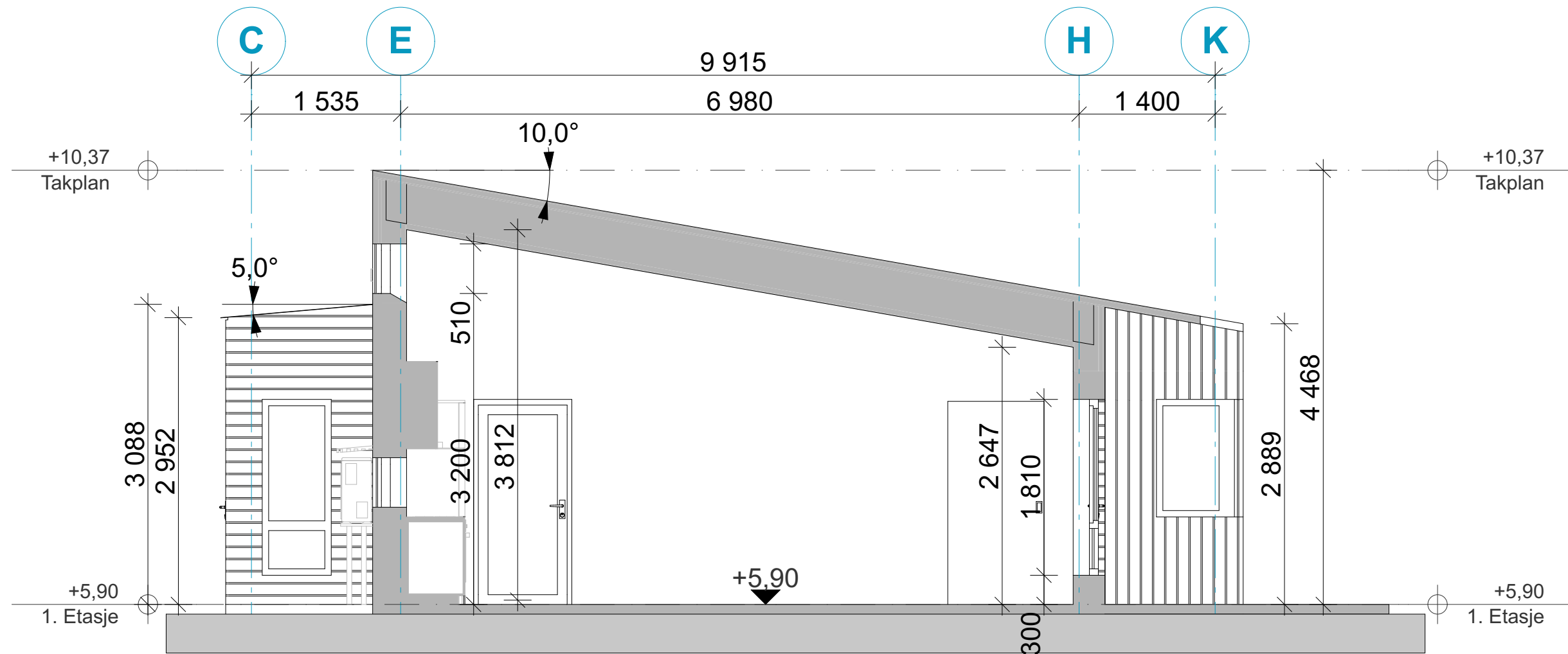
Snitt A 1:50
