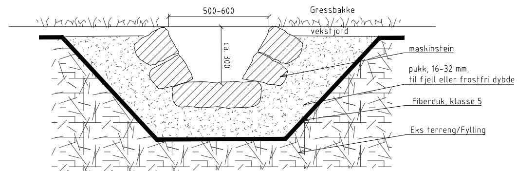
SNITT - Plastret bekkeløp 1:10
