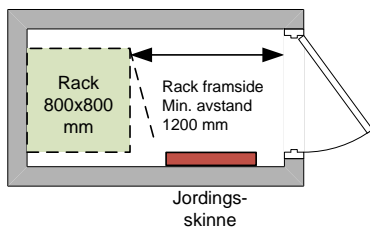
Eksempel på innredning av mindre tekniskrom/nisje hvor kravet til fri plass bak skap avvikes.
