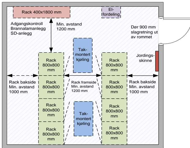
Eksempel på innredning av tekniskrom.
