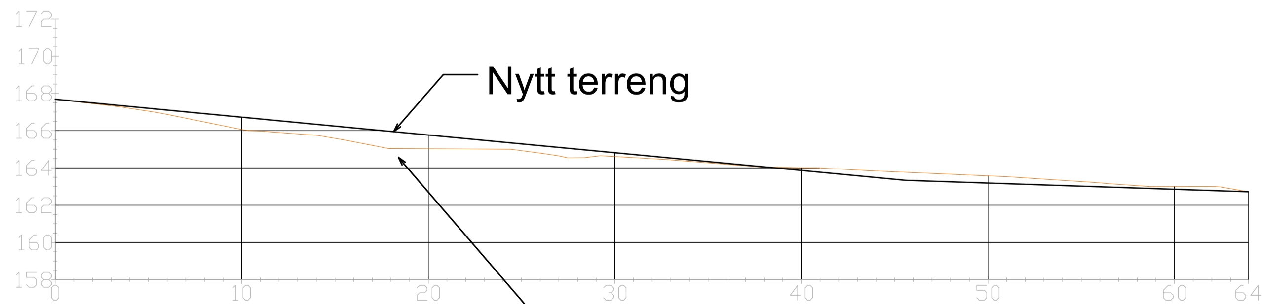
1:200 Stipprofil
