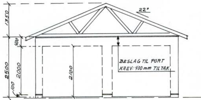
SNITT GARASJE 6x6 OG 6x8M 22°TAK MÅL = 1:50
