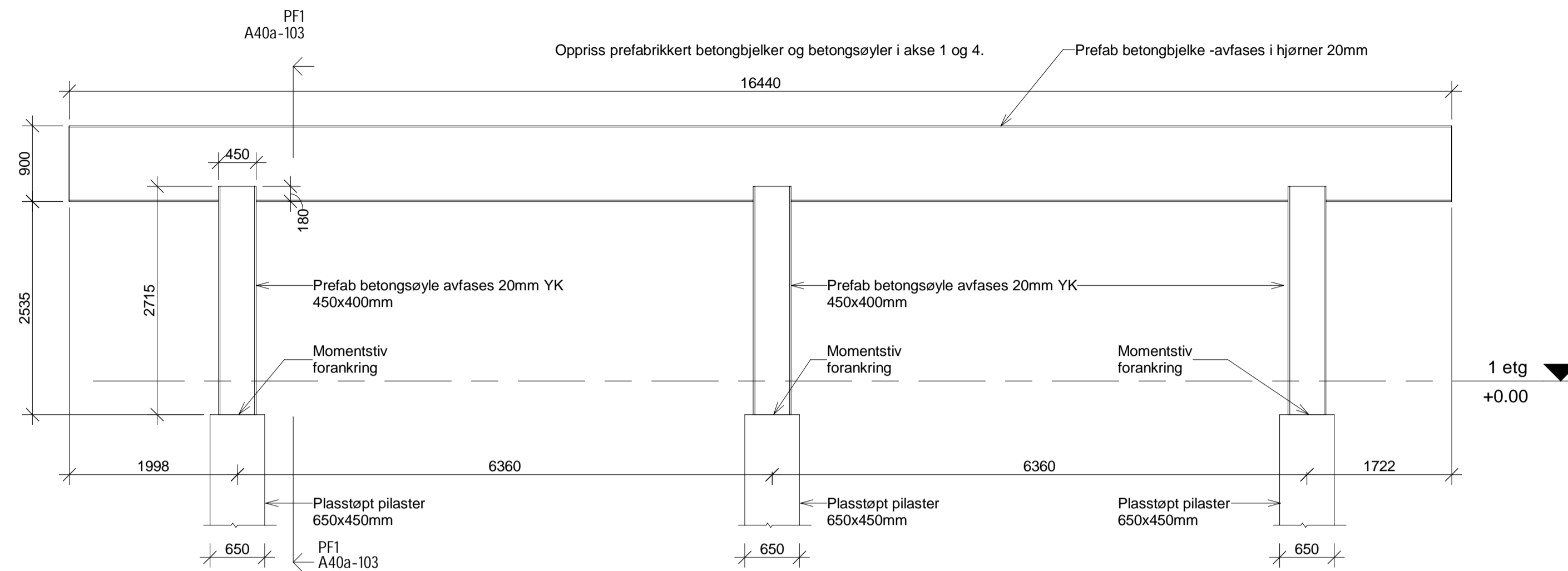
Oppriss prefab bjelke og søyle 1 : 50
