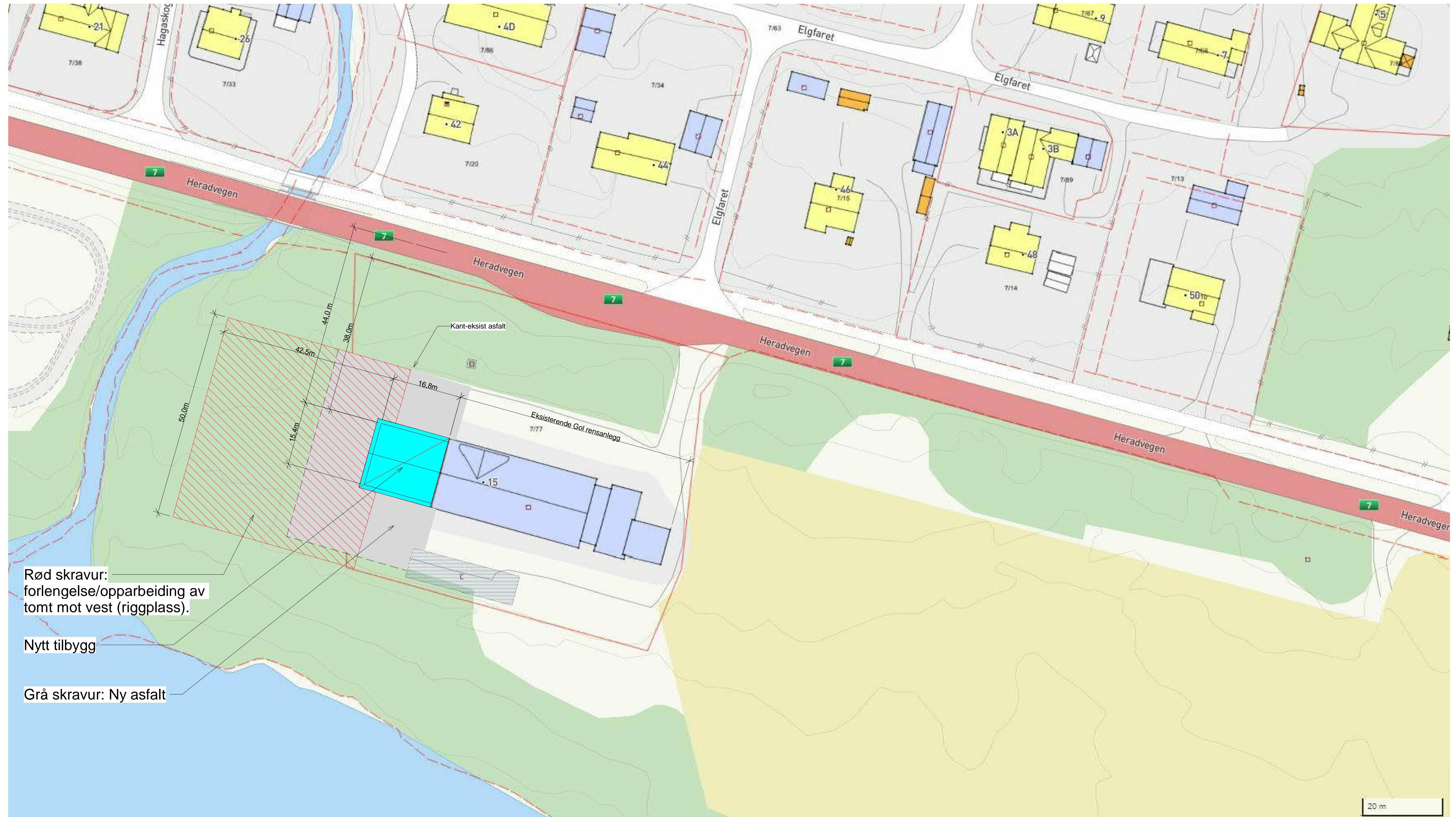
Situasjonsplan 1:500
