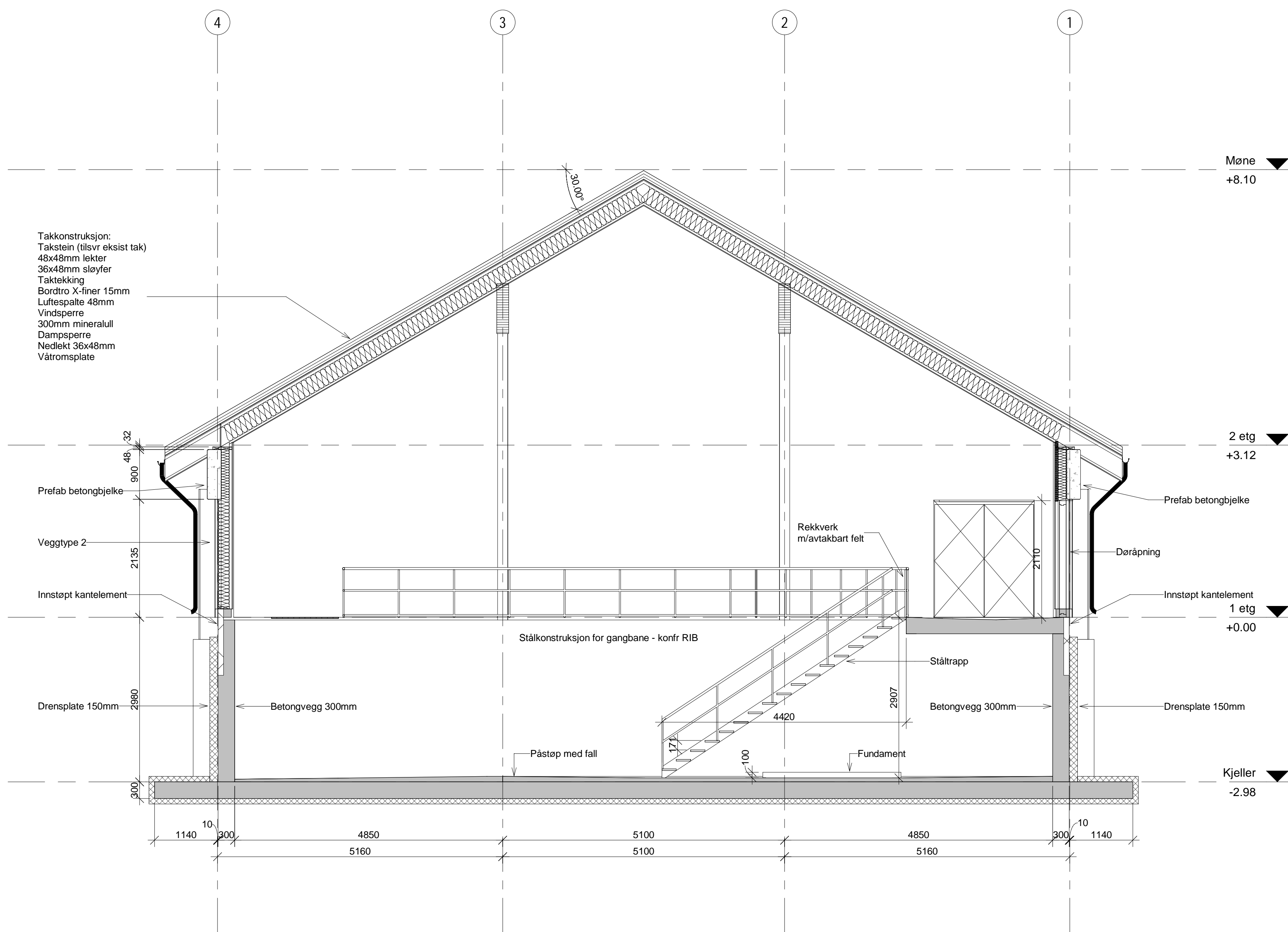
Snitt C 1:50
