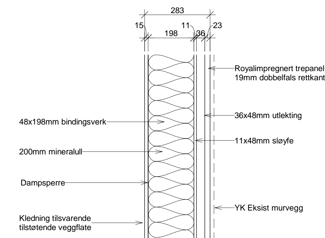
Veggtype 8
