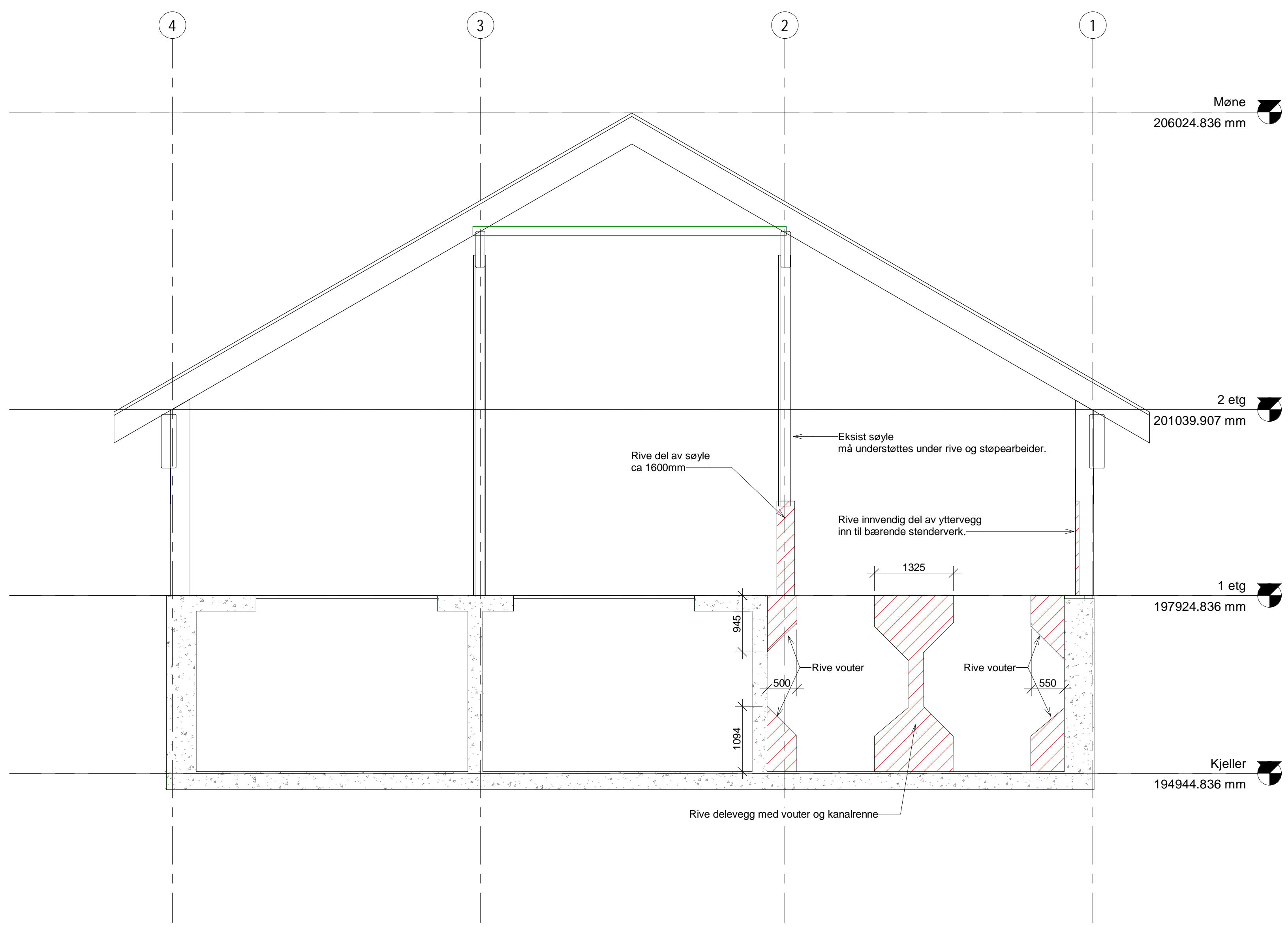
R1 1:50
