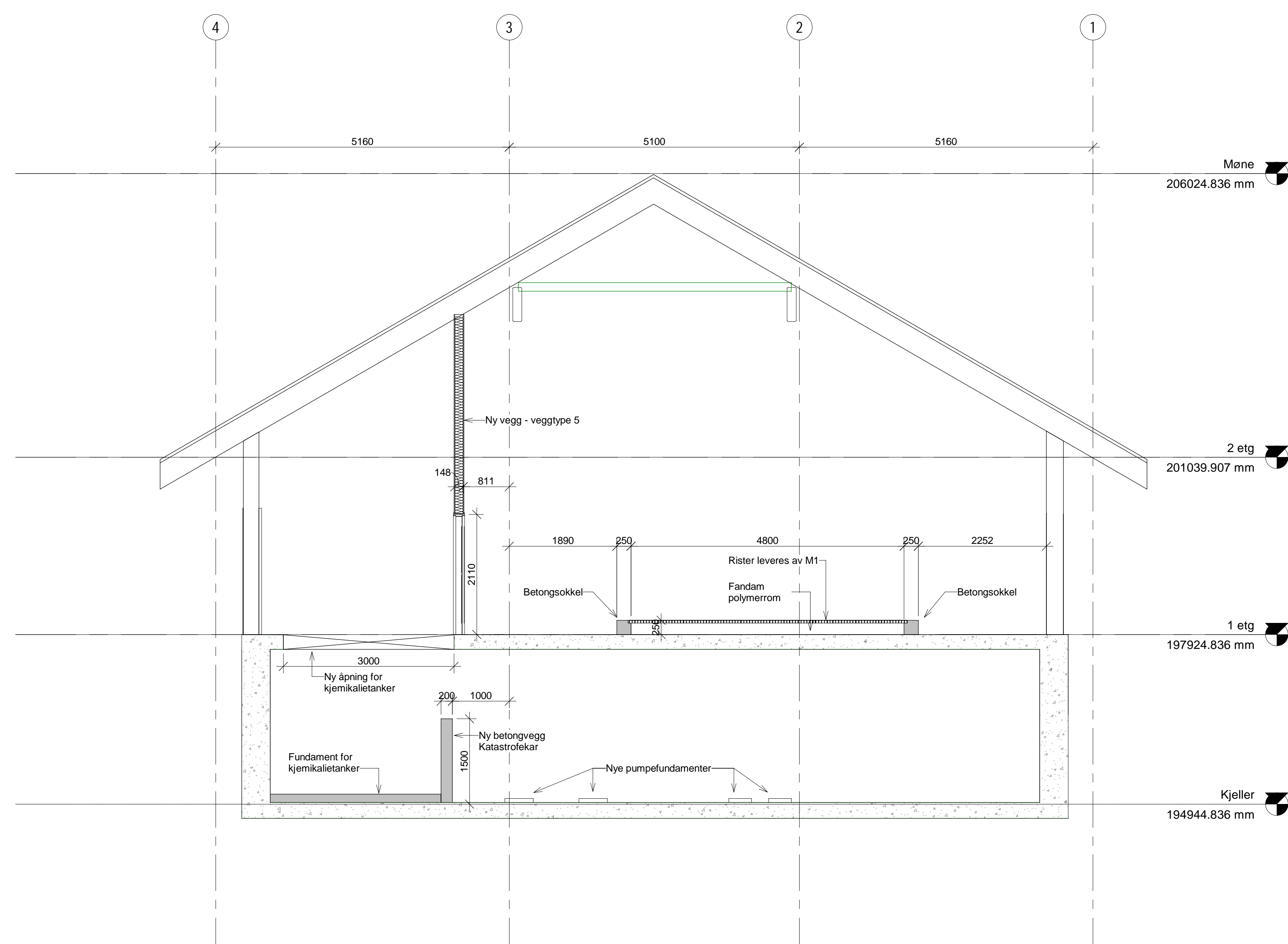
Snitt F 1:50
