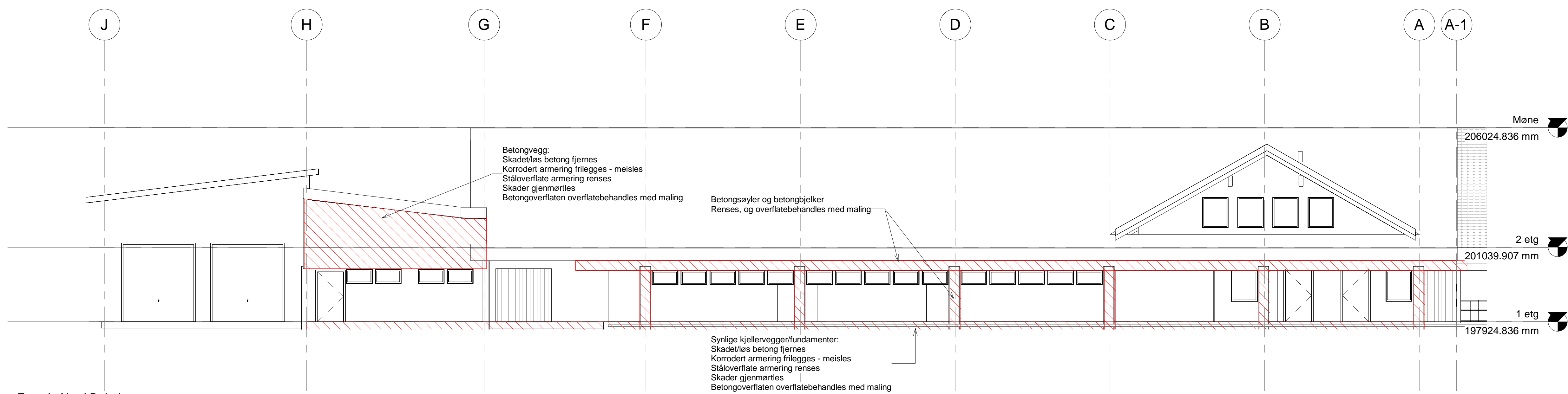
Fasade Nord Rehab 1 : 100
