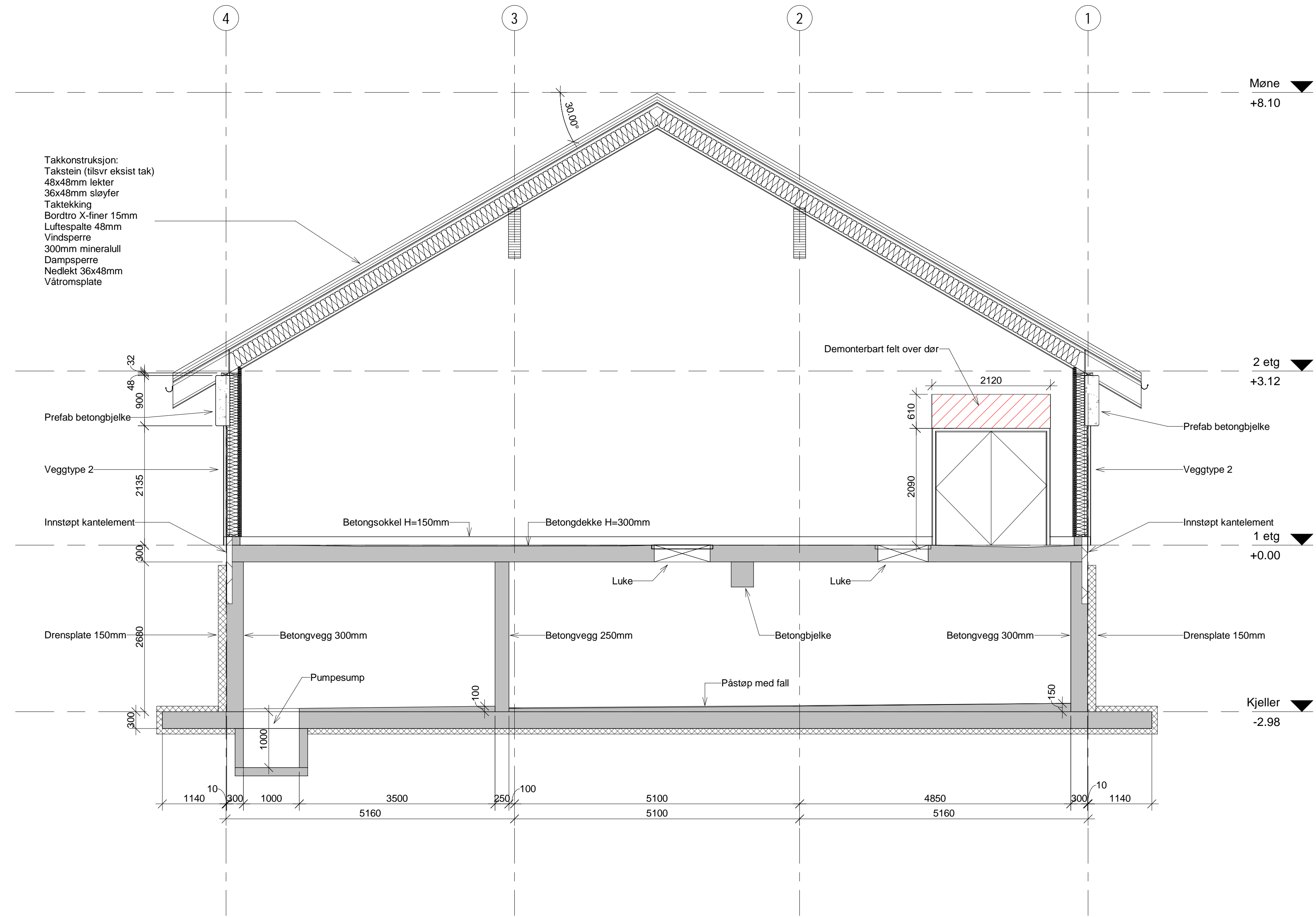
Snitt B 1:50
