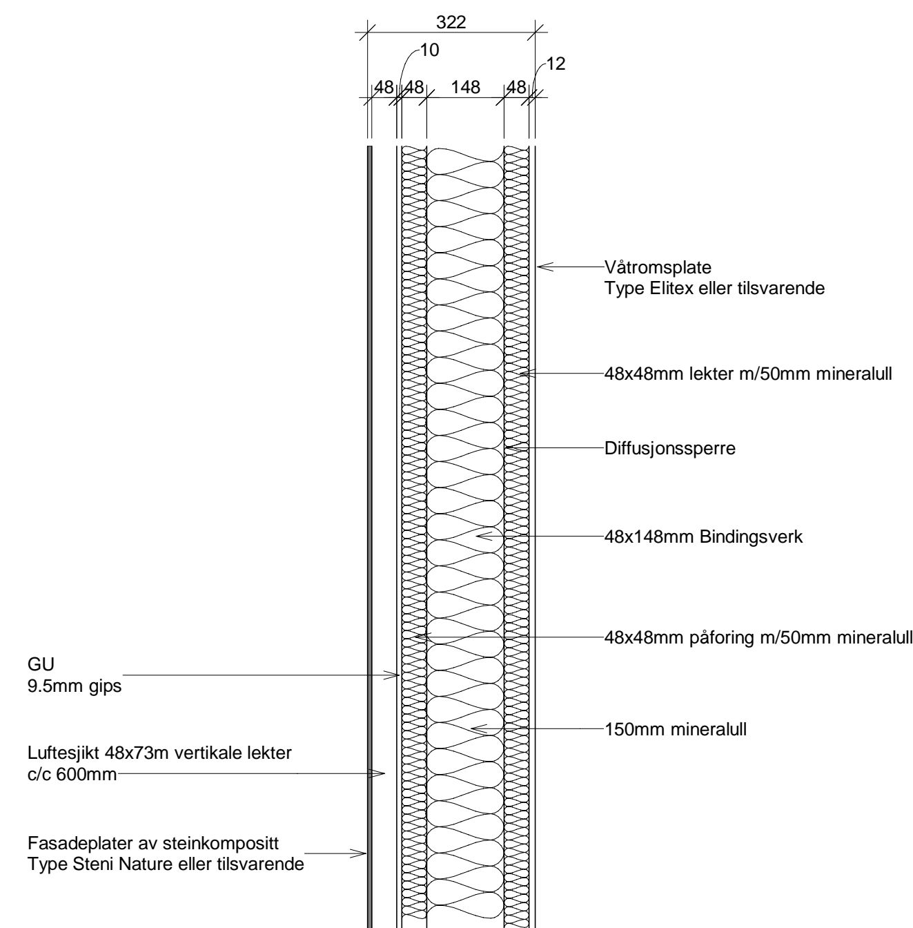
Veggtype 2
