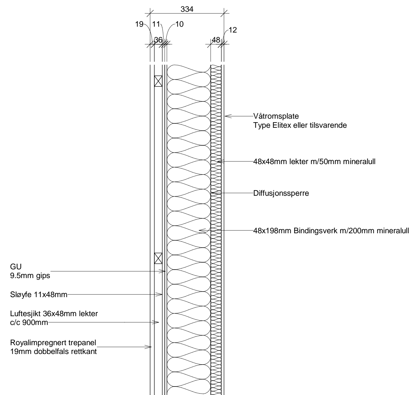
Veggtype 4
