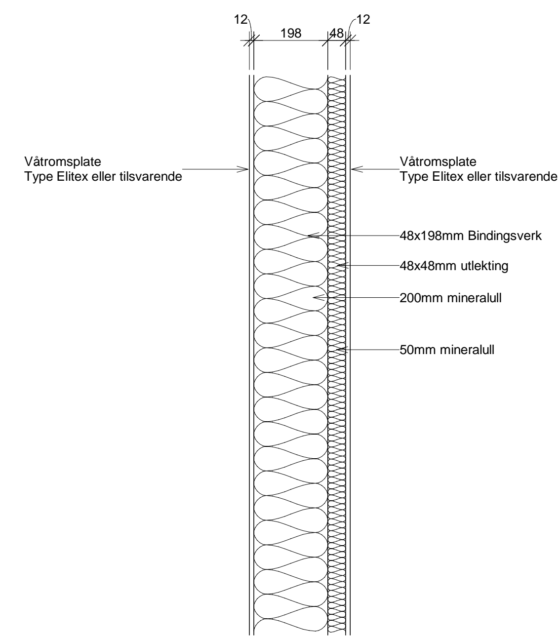
Veggtype 6
