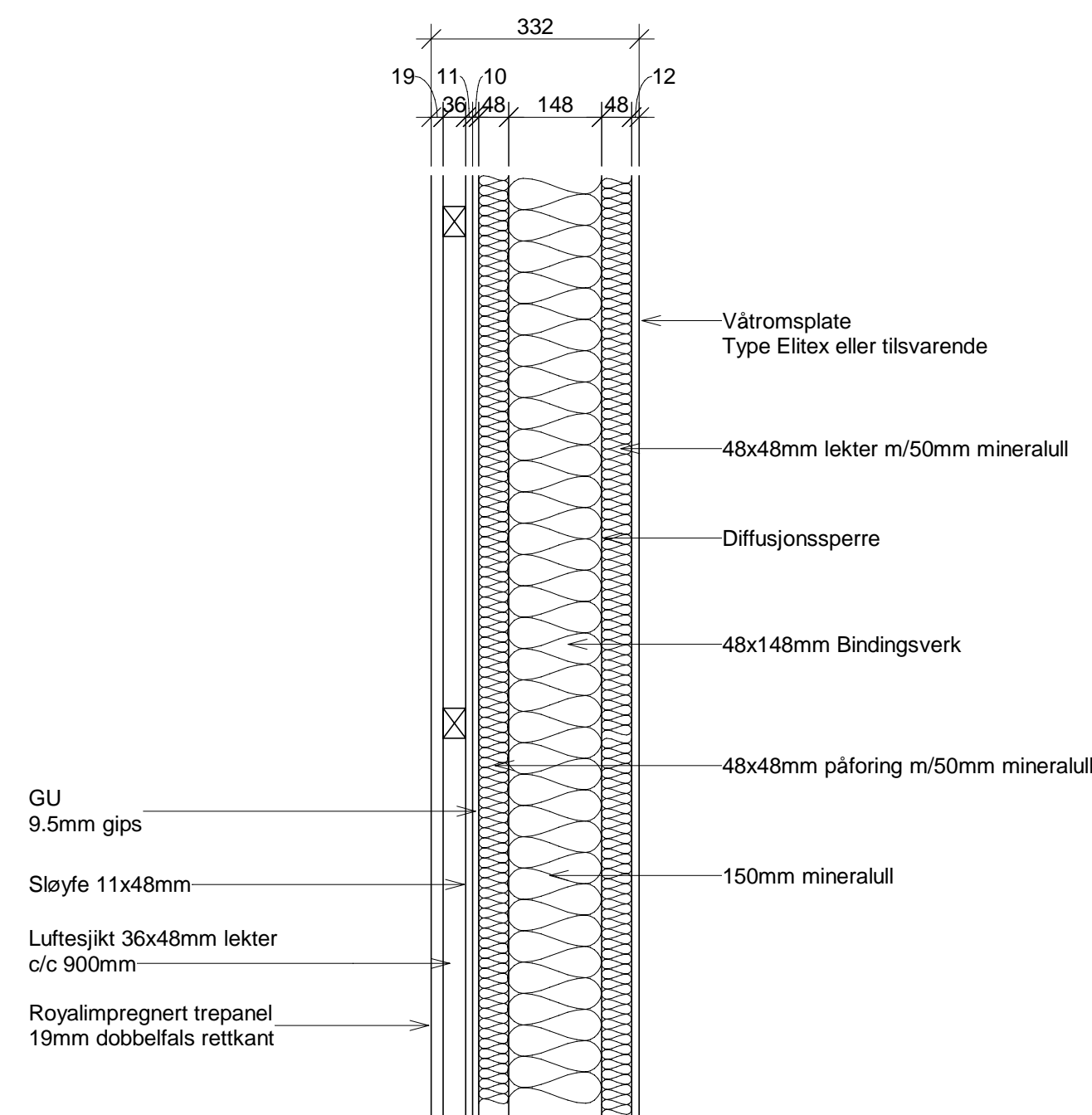
Veggtype 1
