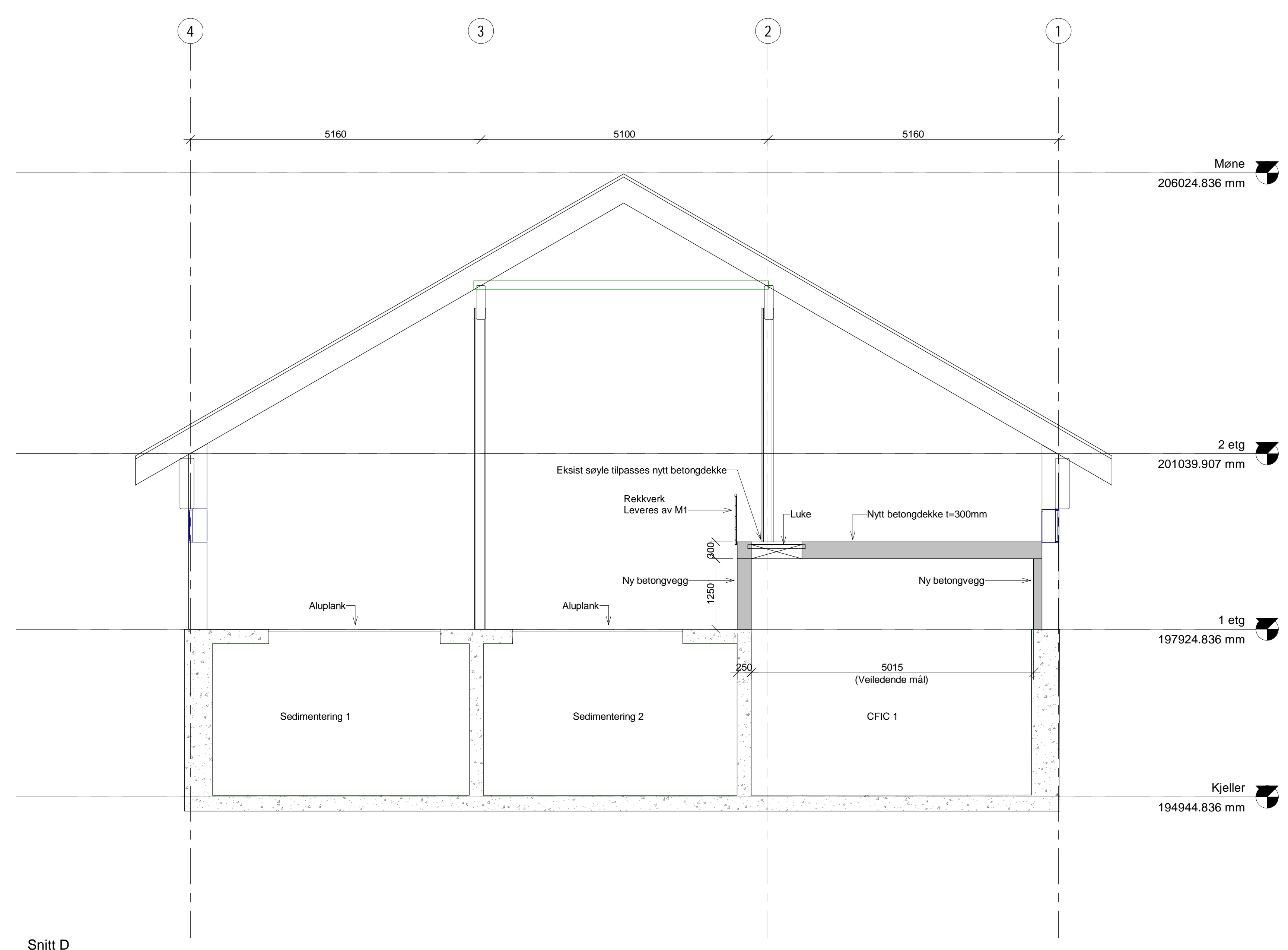
Snitt D 1:50
