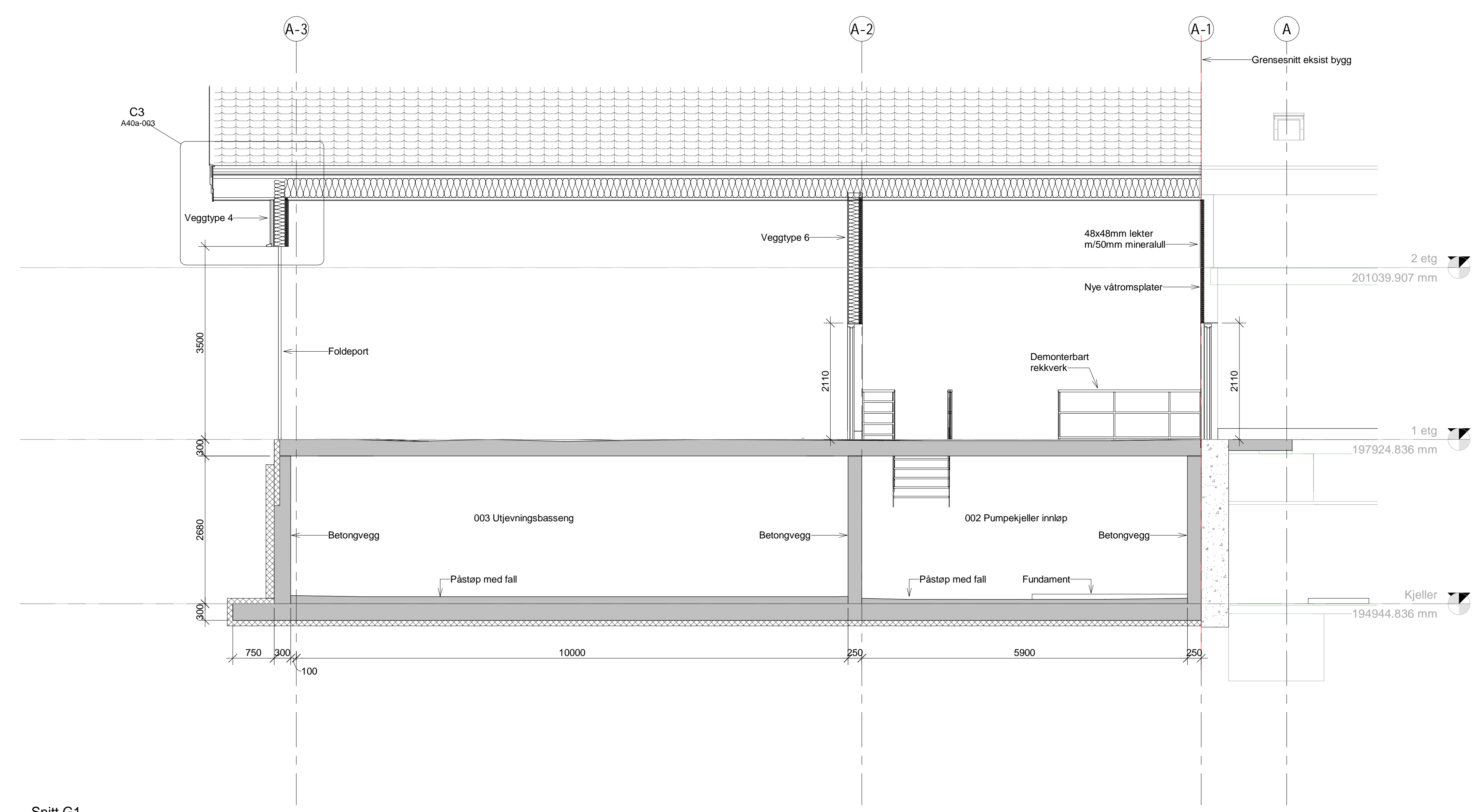
Snitt G1 1:50
