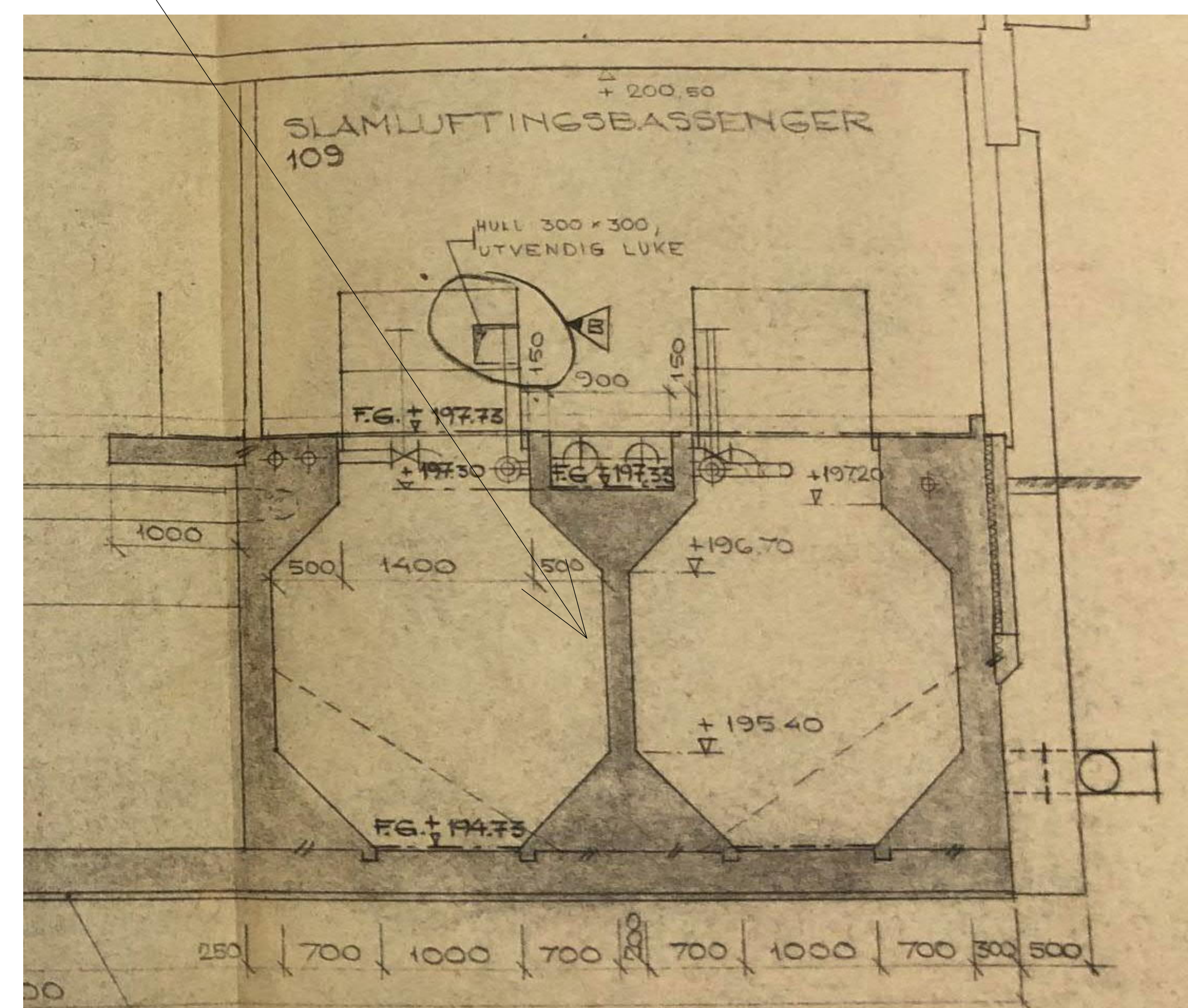
Opprinnelig snitt av bassengvegg som viser vouter og kanal som skal rives.
