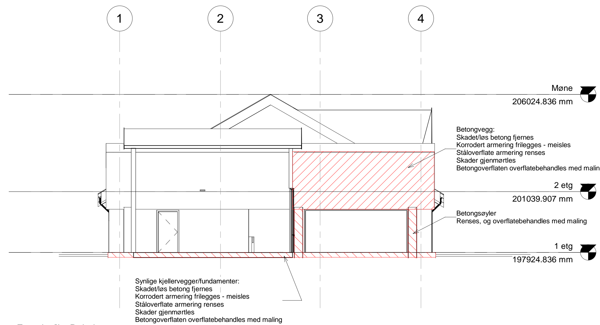
Fasade Øst Rehab 1 : 100
