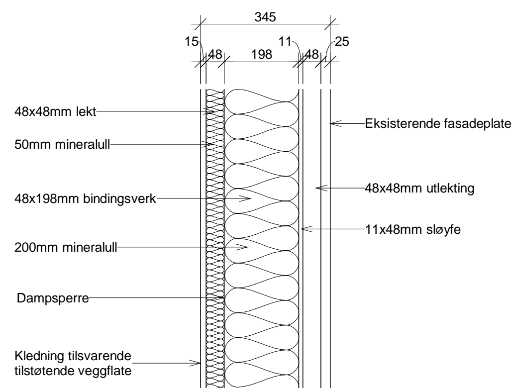
Veggtype 7
