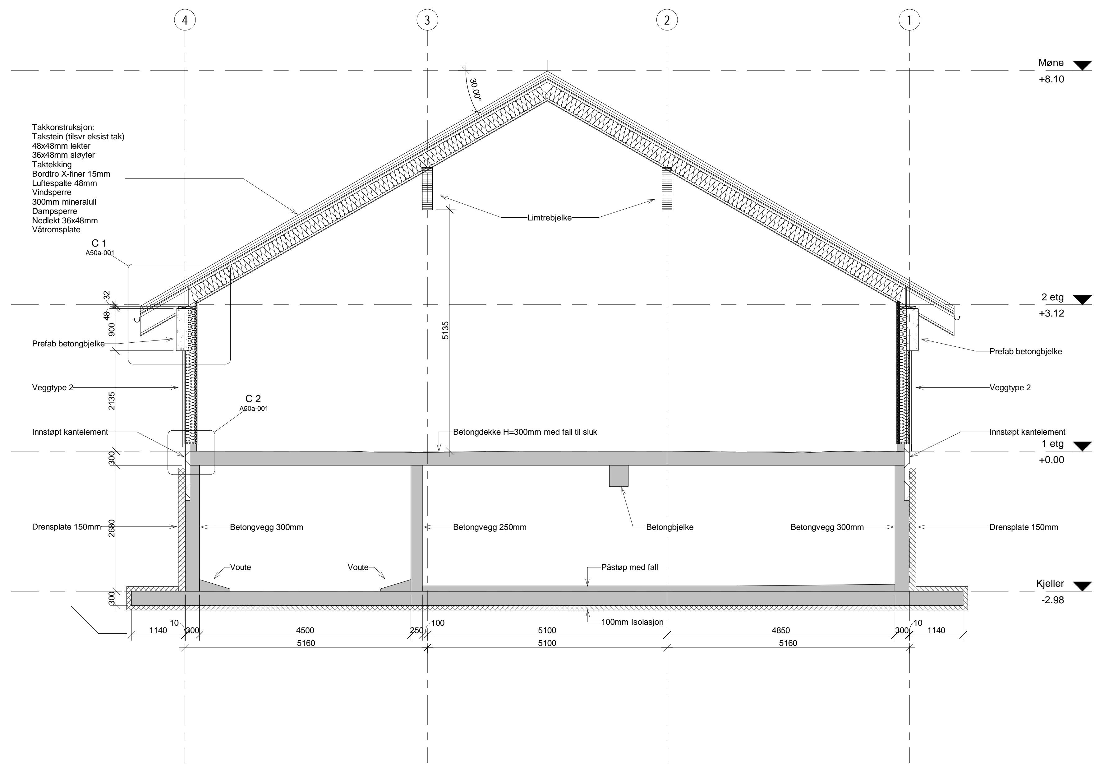
Snitt A 1:50
