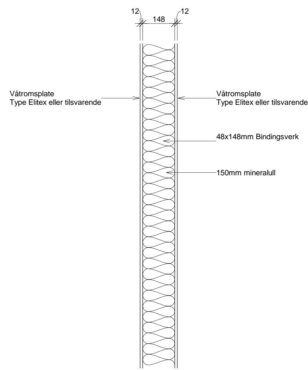
Veggtype 5
