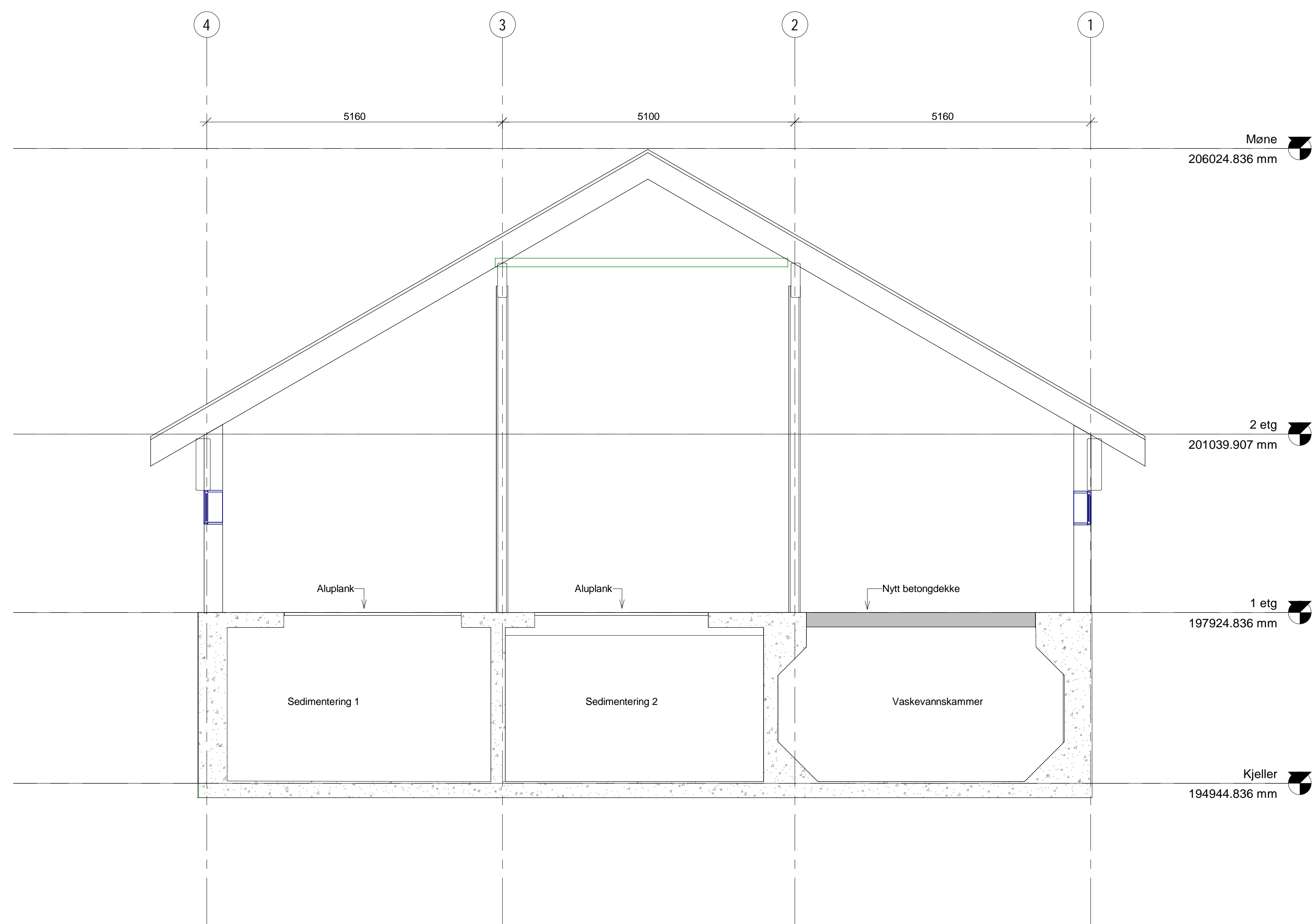
Snitt E 1:50
