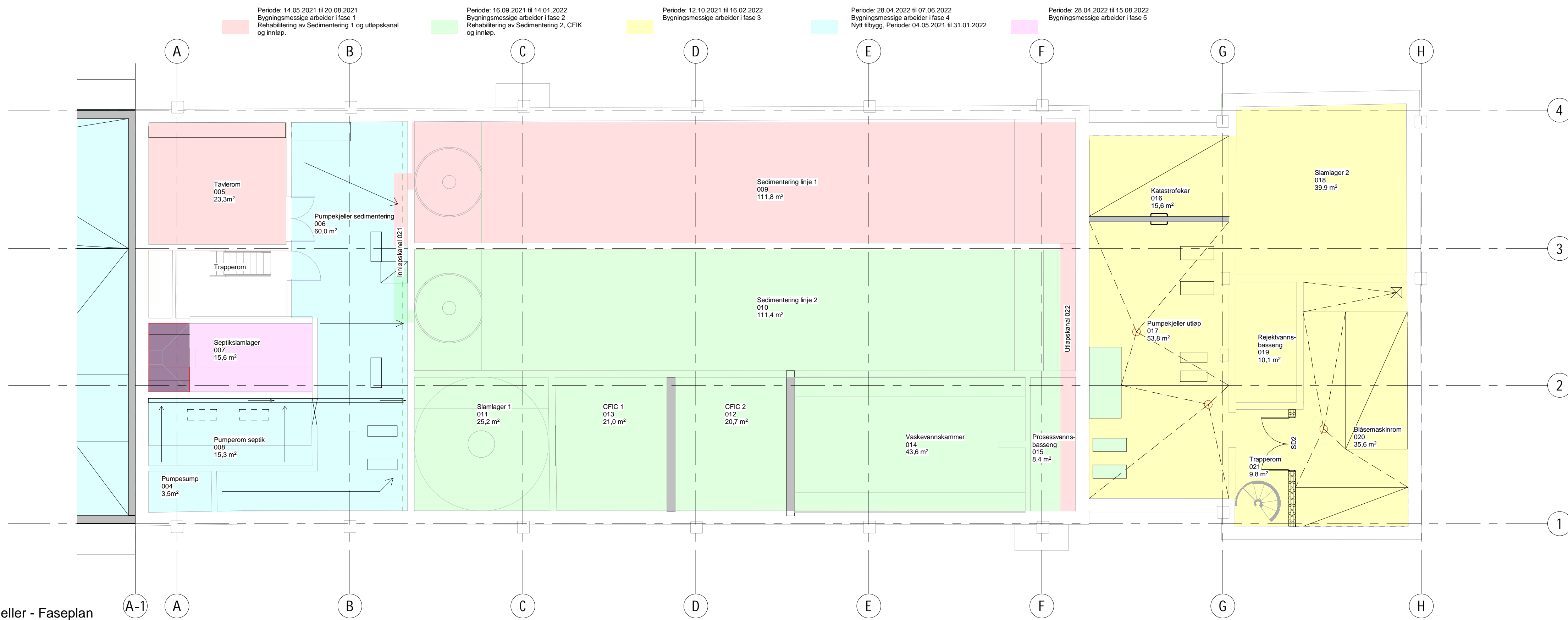
Plan eksist kjeller - Faseplan 1 : 100
