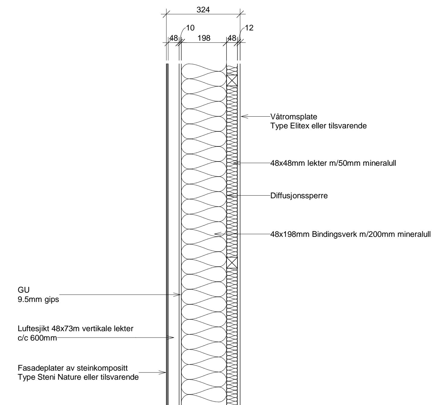
Veggtype 3
