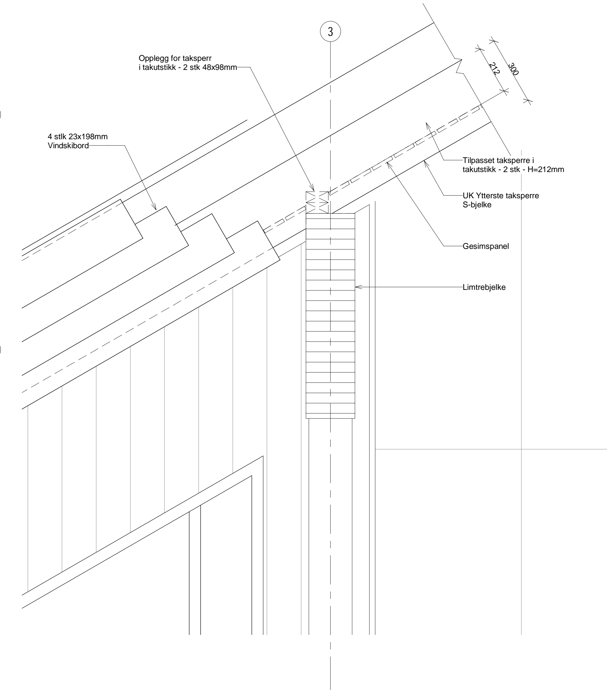
VS3 1:10
