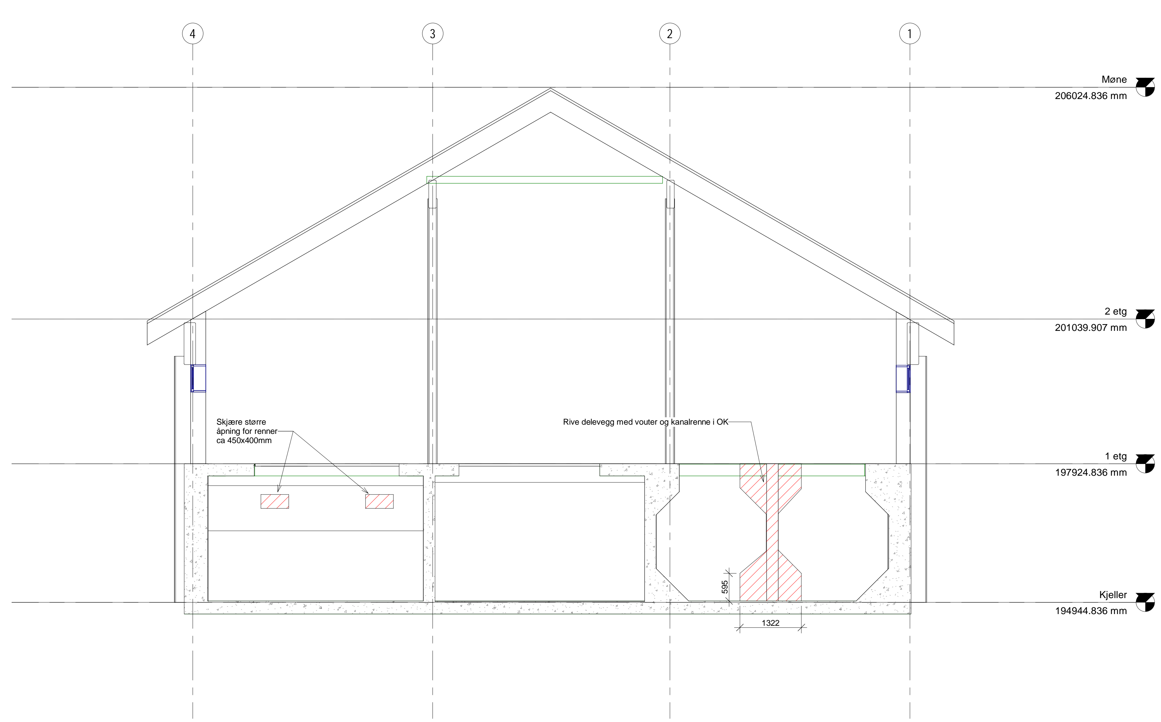
R2 1:50
