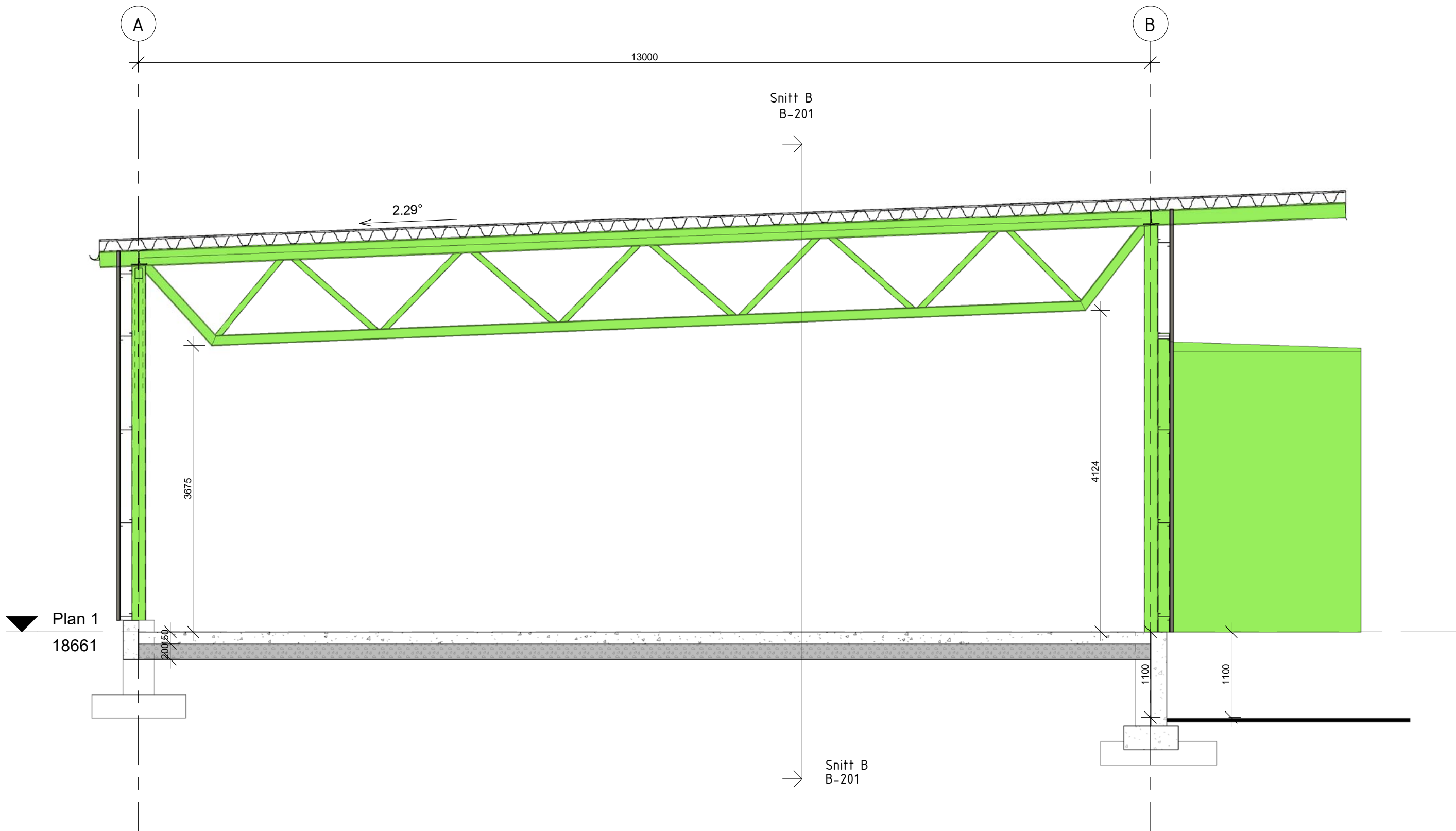
Snitt A 1 : 50
