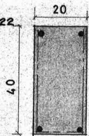
SNITT I DRAGER 5 M:1:10
