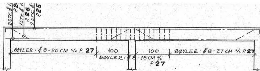
OPDRISS AV DRAGER 1 H/B=40/25
