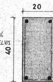
SNITT I DRAGER 2 M:1:10
