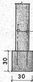
SØYLEFUNDAMENT 3 M:1:20
