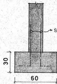
SØYLEFUNDAMENT 2 M:1:20
