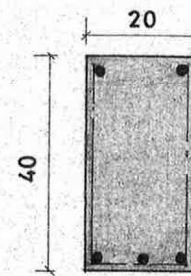
SNITT I D. 1 M:1:10
