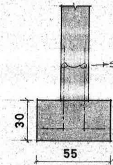
SØYLEFUNDAMENT 1 M:1:20
