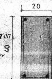
SNITT I DRAGER 4 M:1:10
