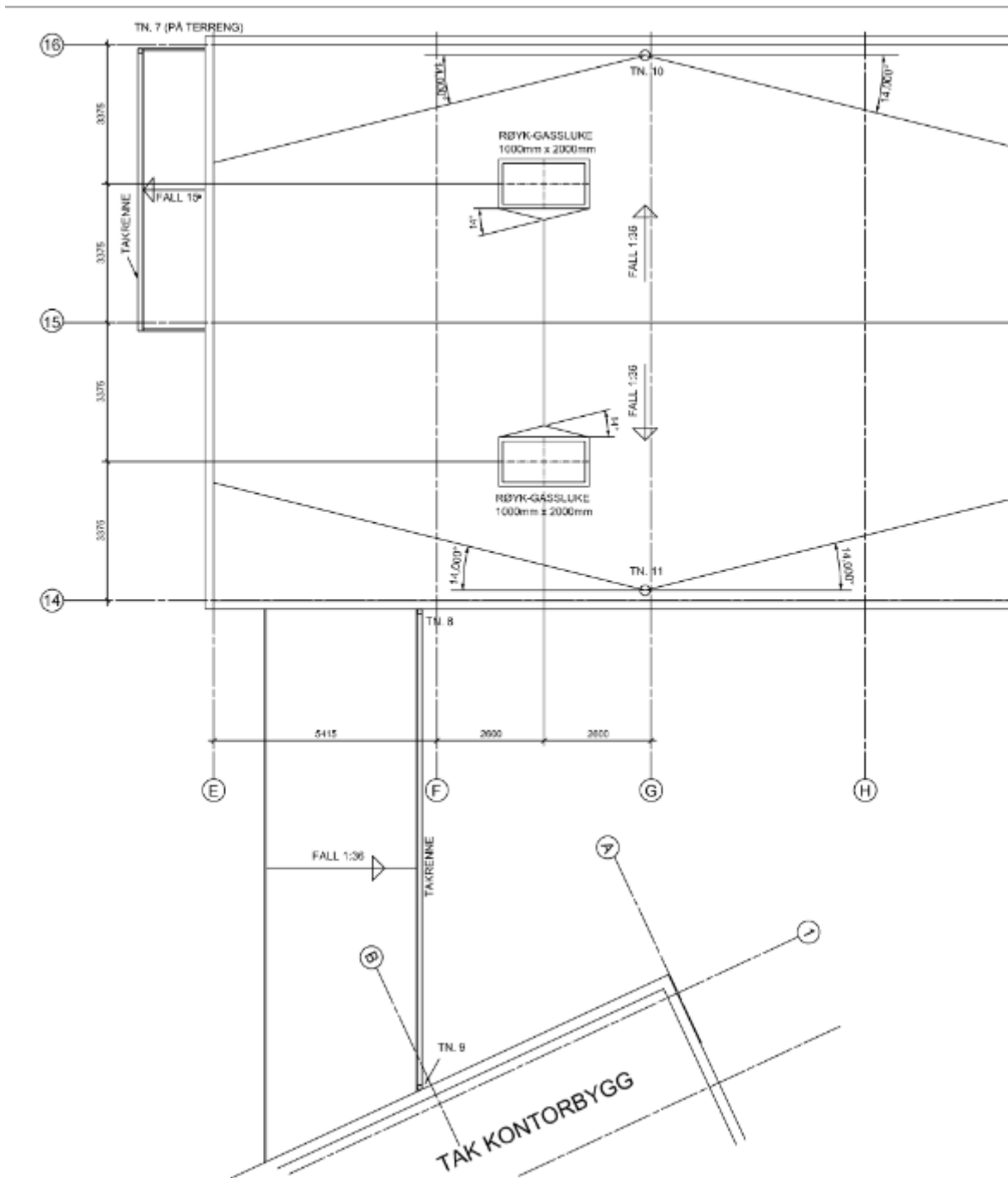
Takplan
