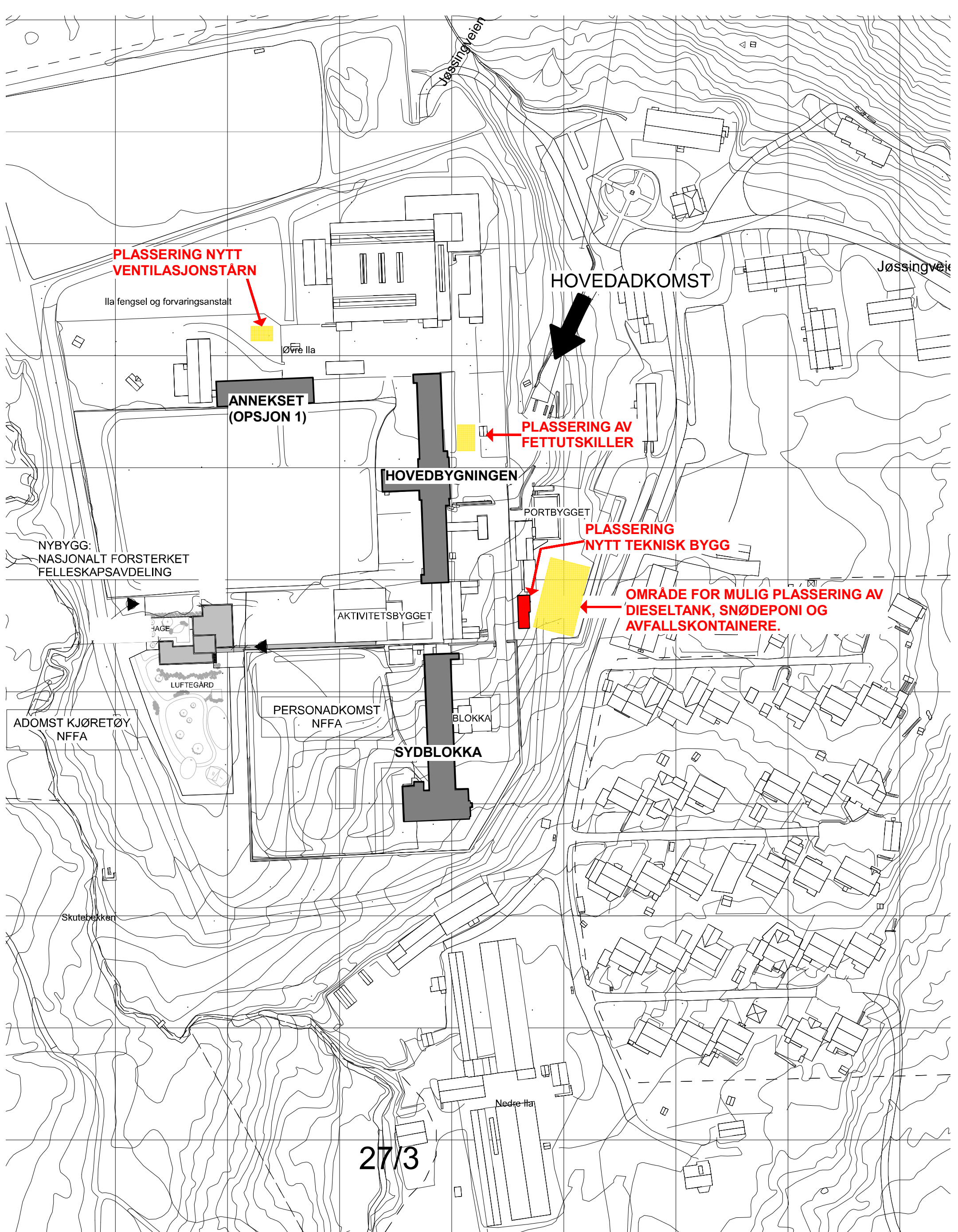
Ila fengsel - rehabilitering av tekniske anlegg. Situasjonsplan med nye tiltak 1:1500 = A3
