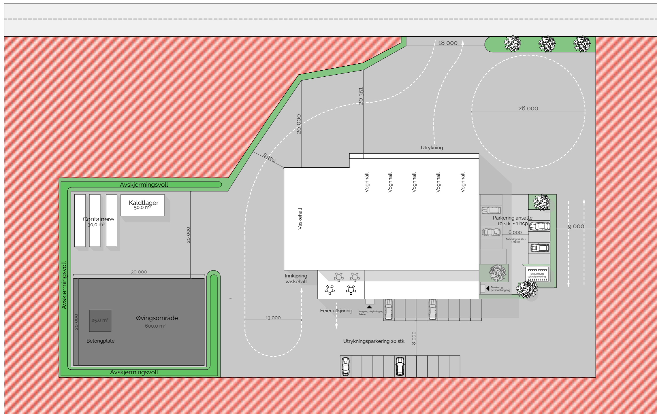
1:500 Utomhusplan
