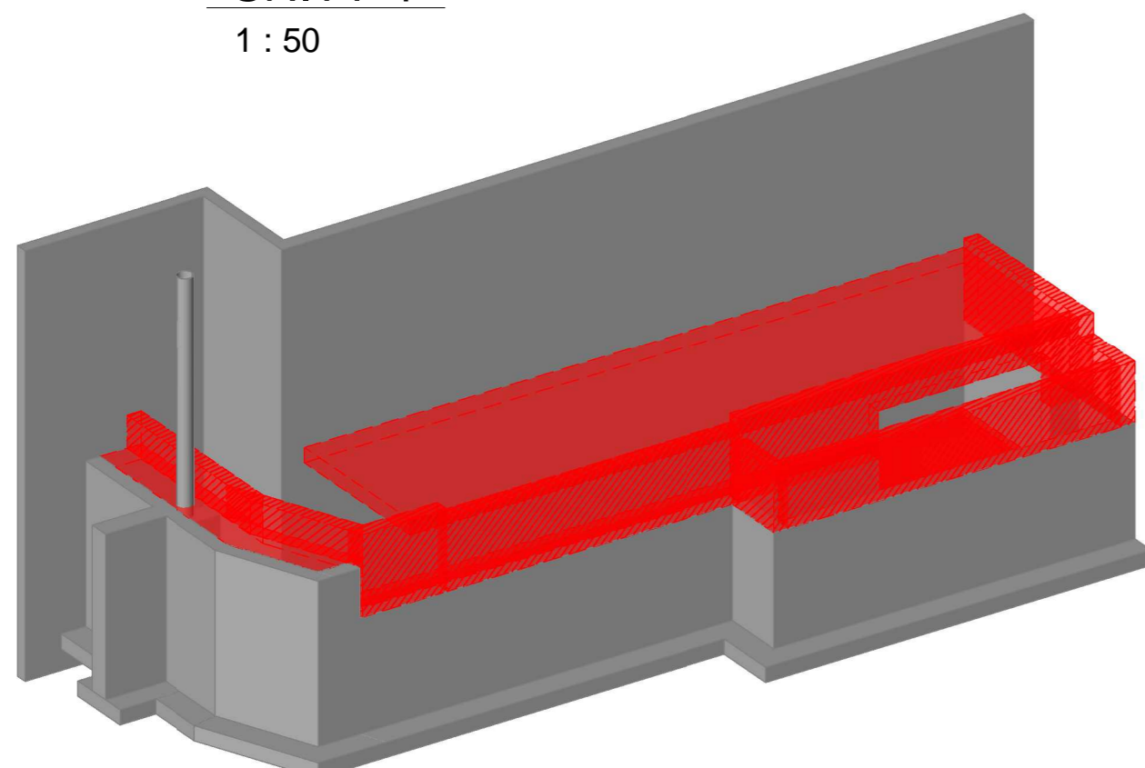
3D Nettstasjon Riving fase C - 1
