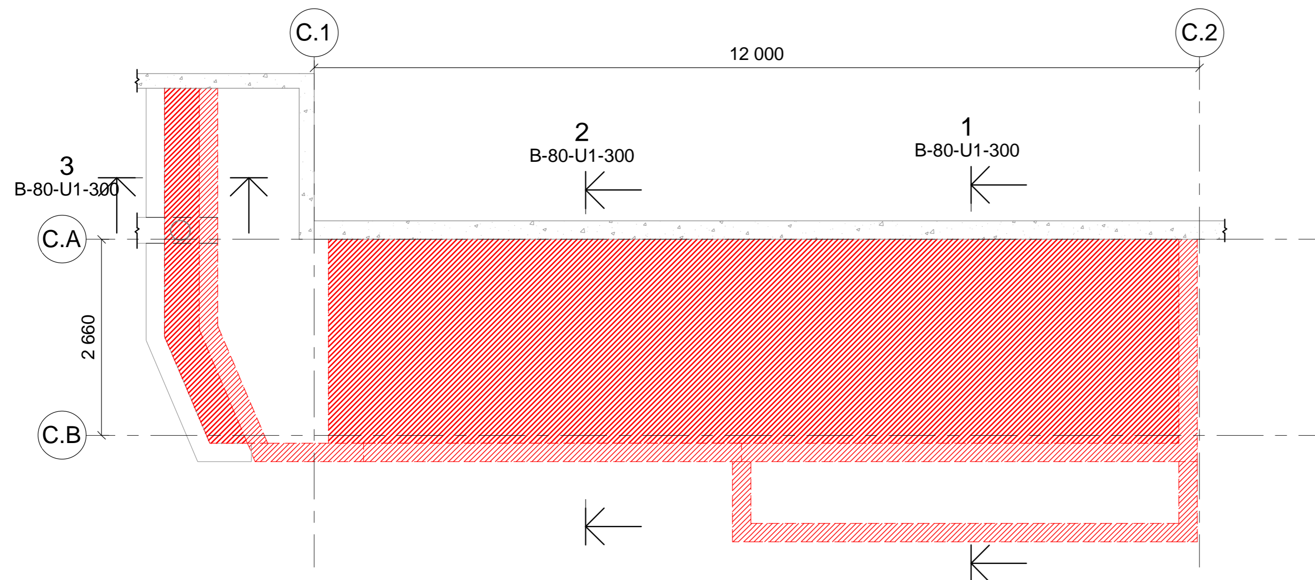
PLAN RIVING U1. ETG - NETTSTASJON FASE C
