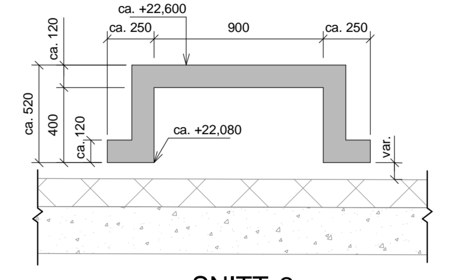
SNITT 2 1 : 20
