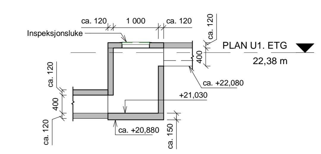
SNITT A 1 : 50
