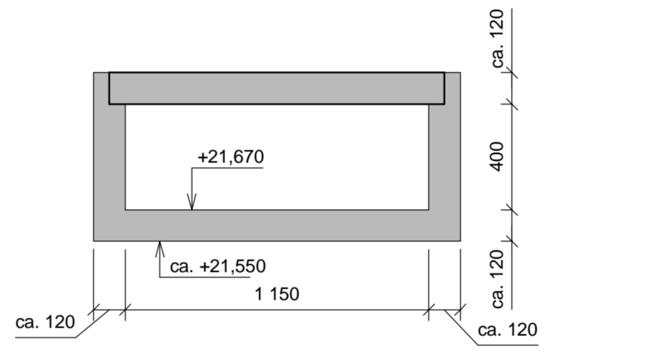
SNITT 3 1 : 20
