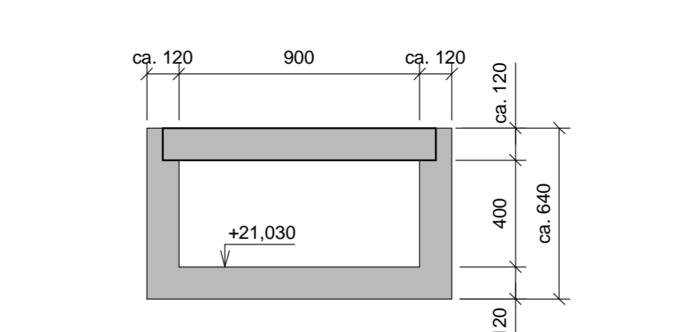
SNITT 1 1 : 20
