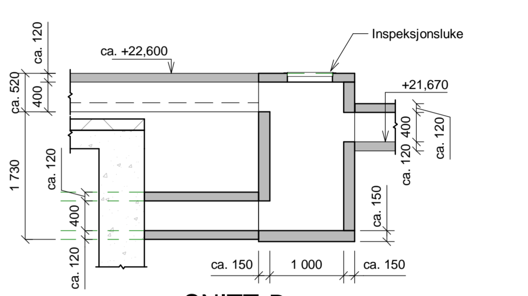
SNITT B 1 : 50
