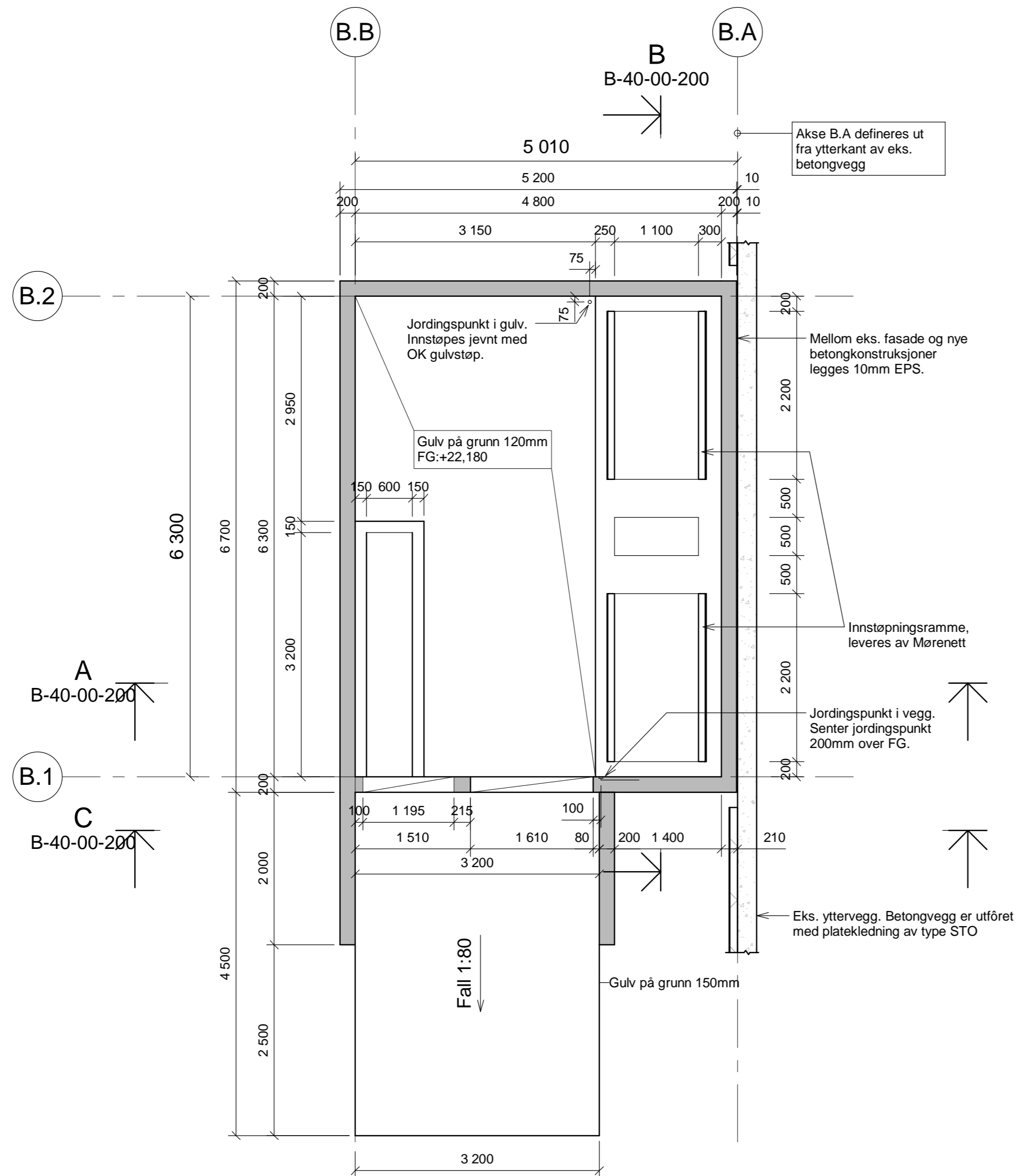
PLAN U1. ETG - NETTSTASJON FASE B 1 : 50
