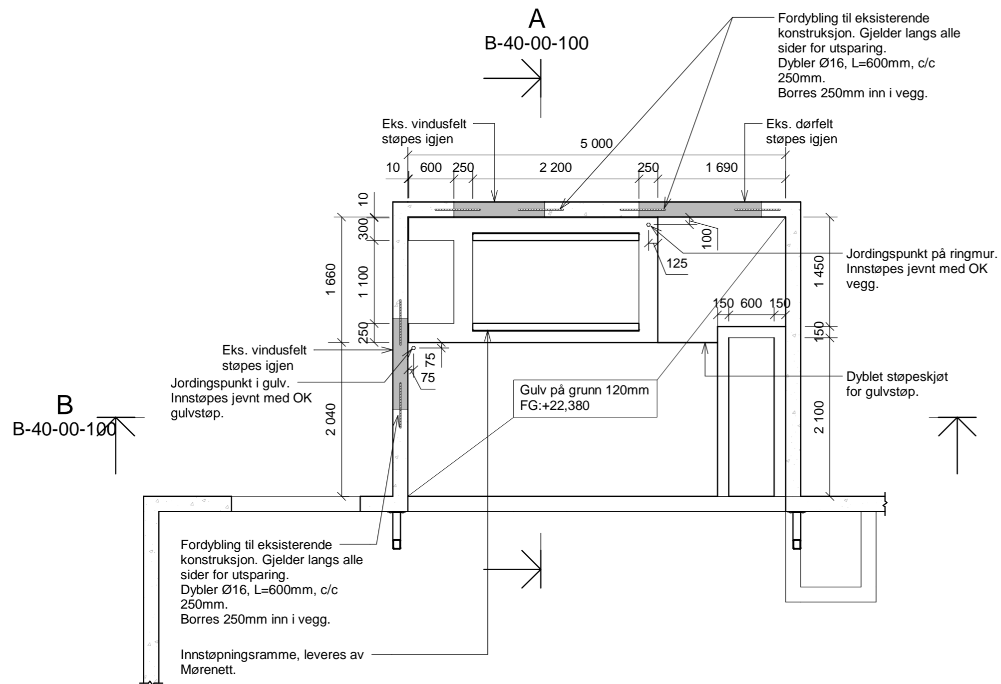
PLAN U1. ETG - NETTSTASJON FASE A
