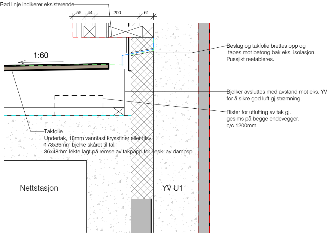
Nettstasjon - Tilslutning til eksisterende YV 1 : 10
