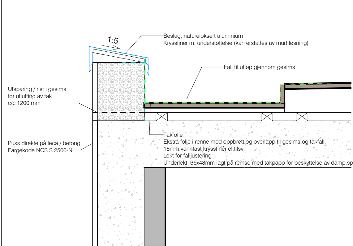
Nettstasjon - Gesims 1 : 10
