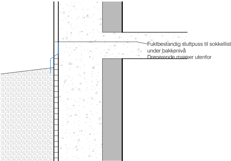
Nettstasjon - Sokkel 1 : 10
