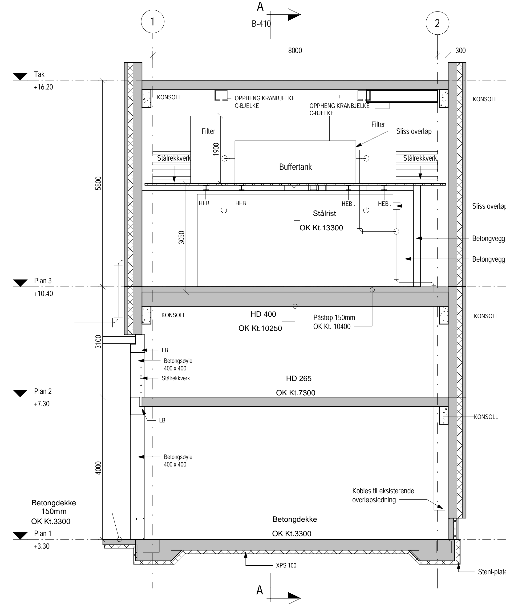
SNITT B-B 1 : 50
