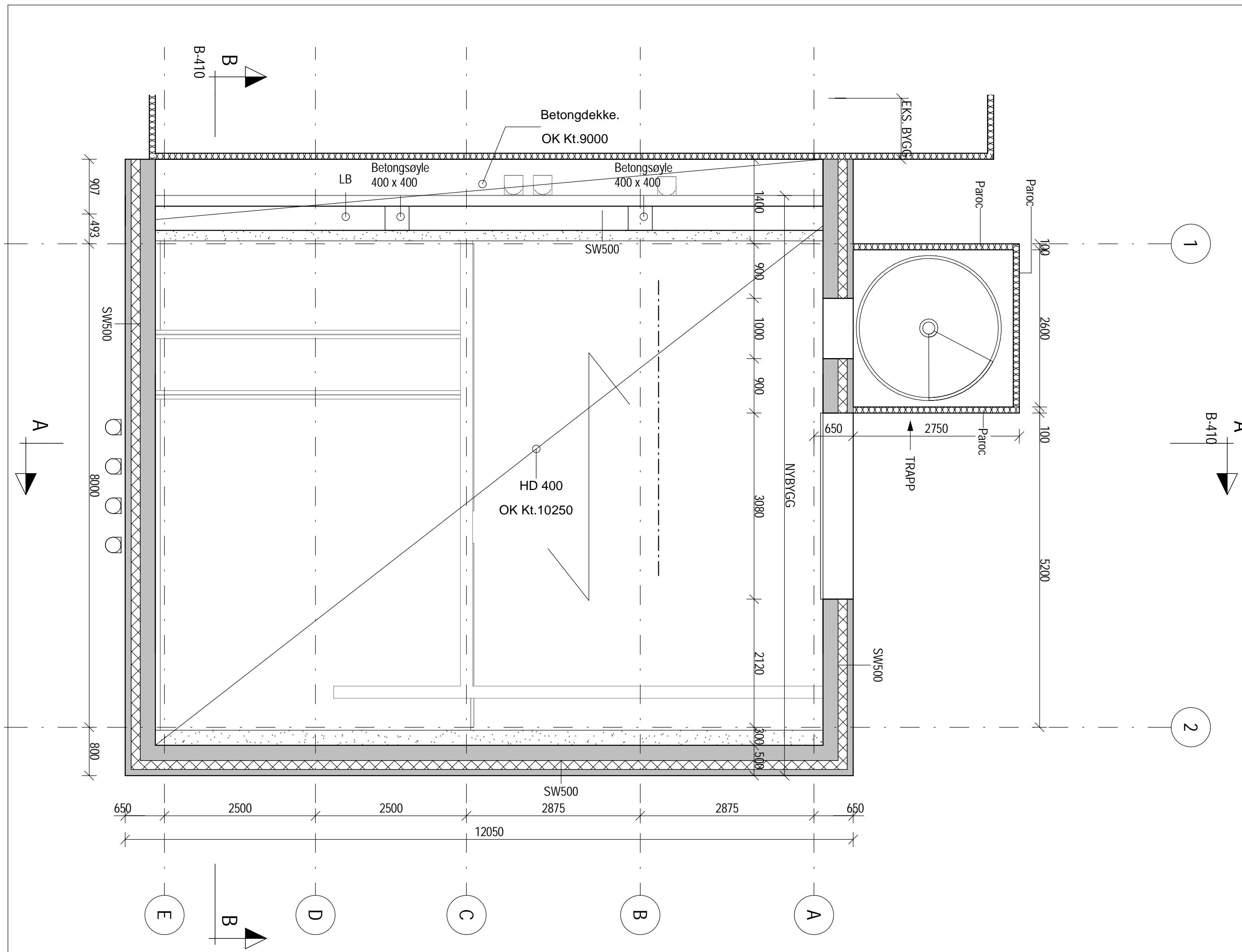
PLAN DEKKE OVER 2. ETG 1:50
