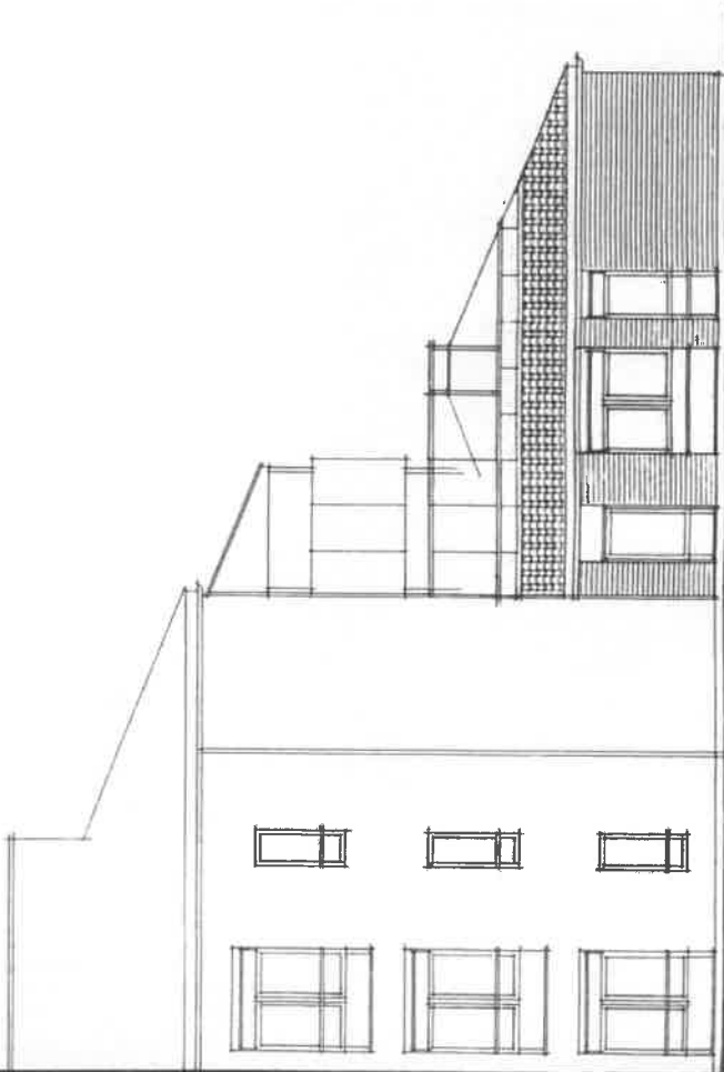
FASADE VEST
