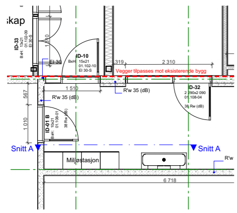
Rom nr. 108 1. Etasje 1:100
