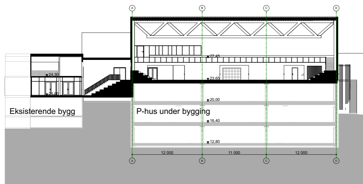
1:400 Snitt B
