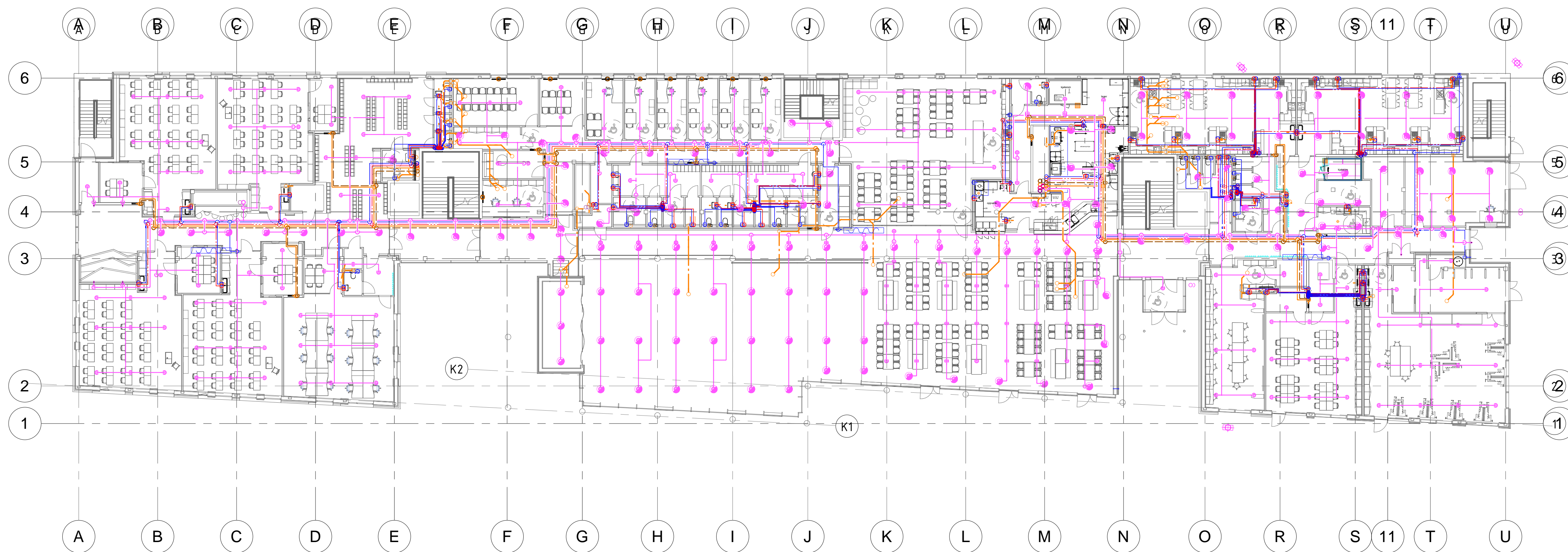
Røranlegg Plan 02 1:200
