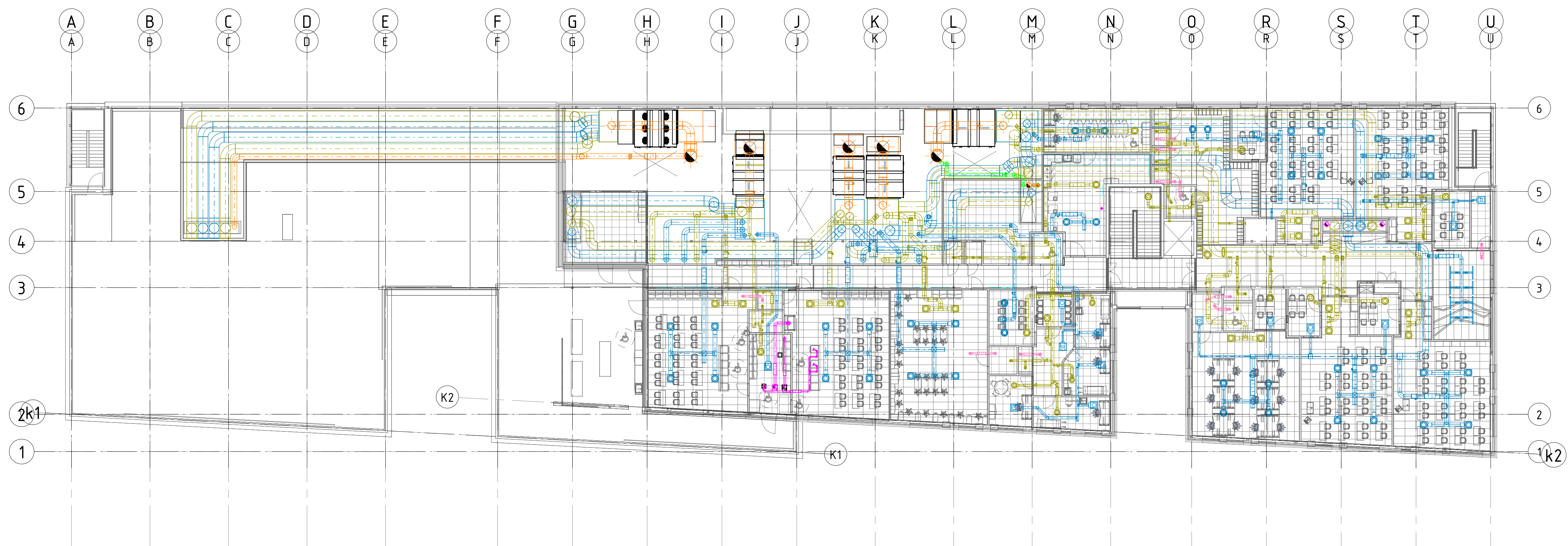
Ventilasjonsanlegg Plan 04 1:200
