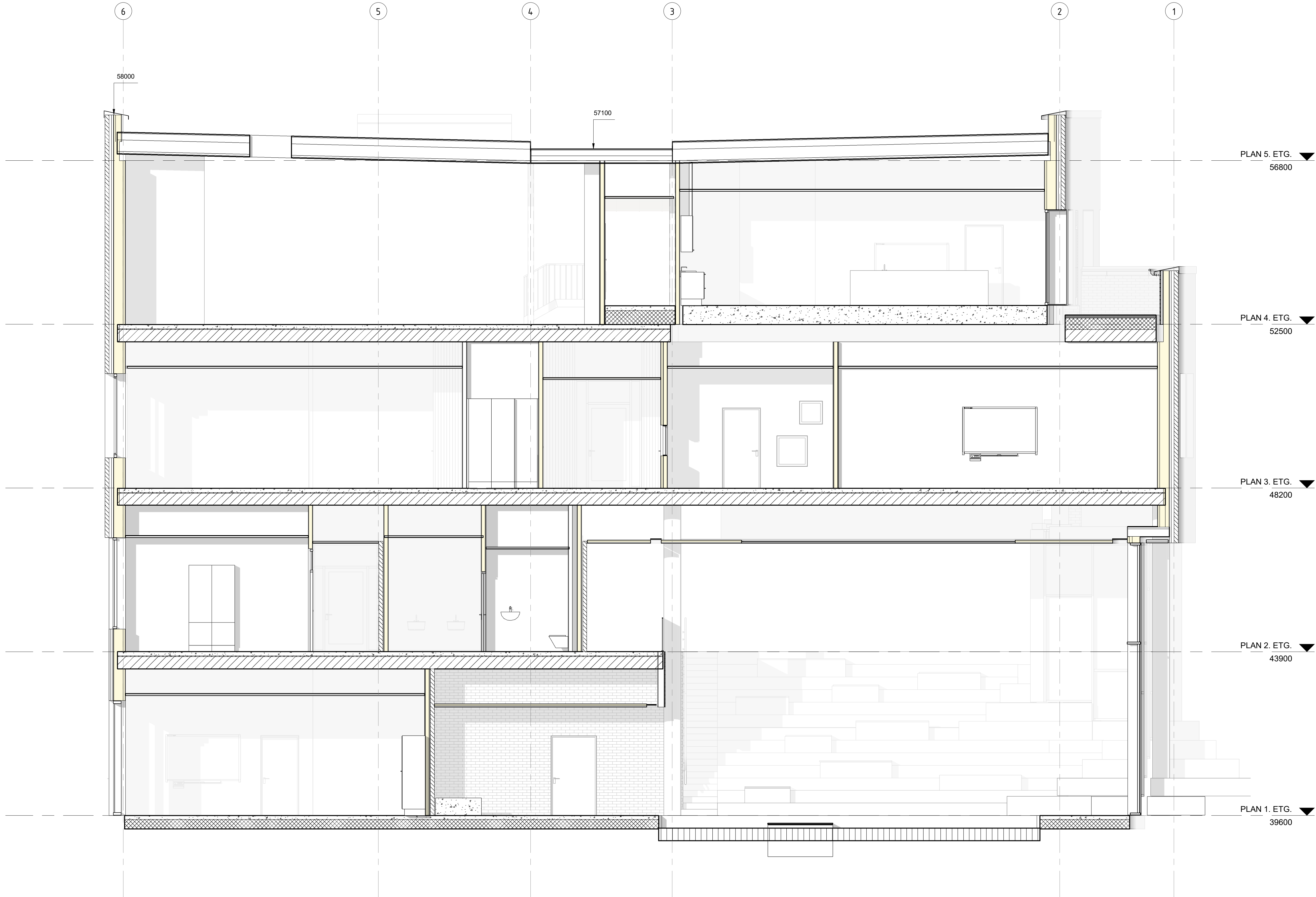
Snitt FF 1-50 1 : 50
