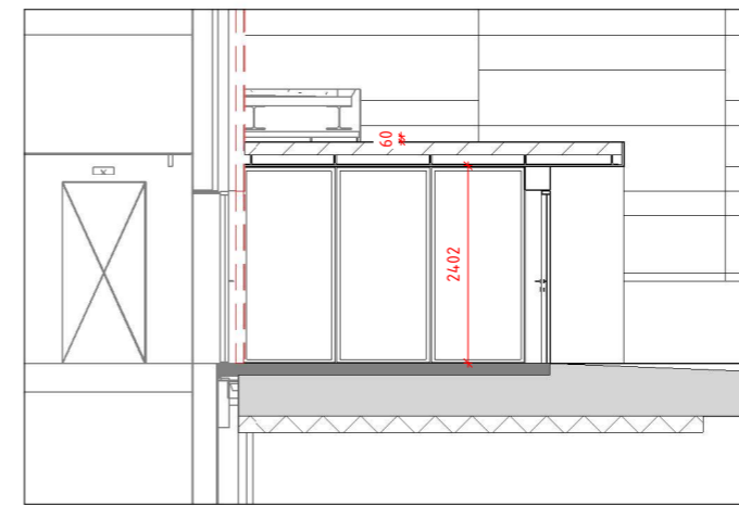
SNITT 1:100
