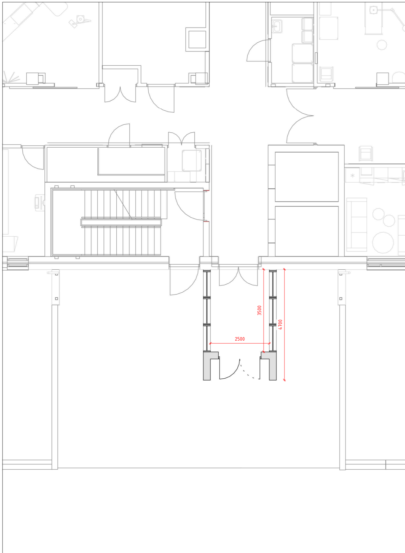
PLAN 1:100
