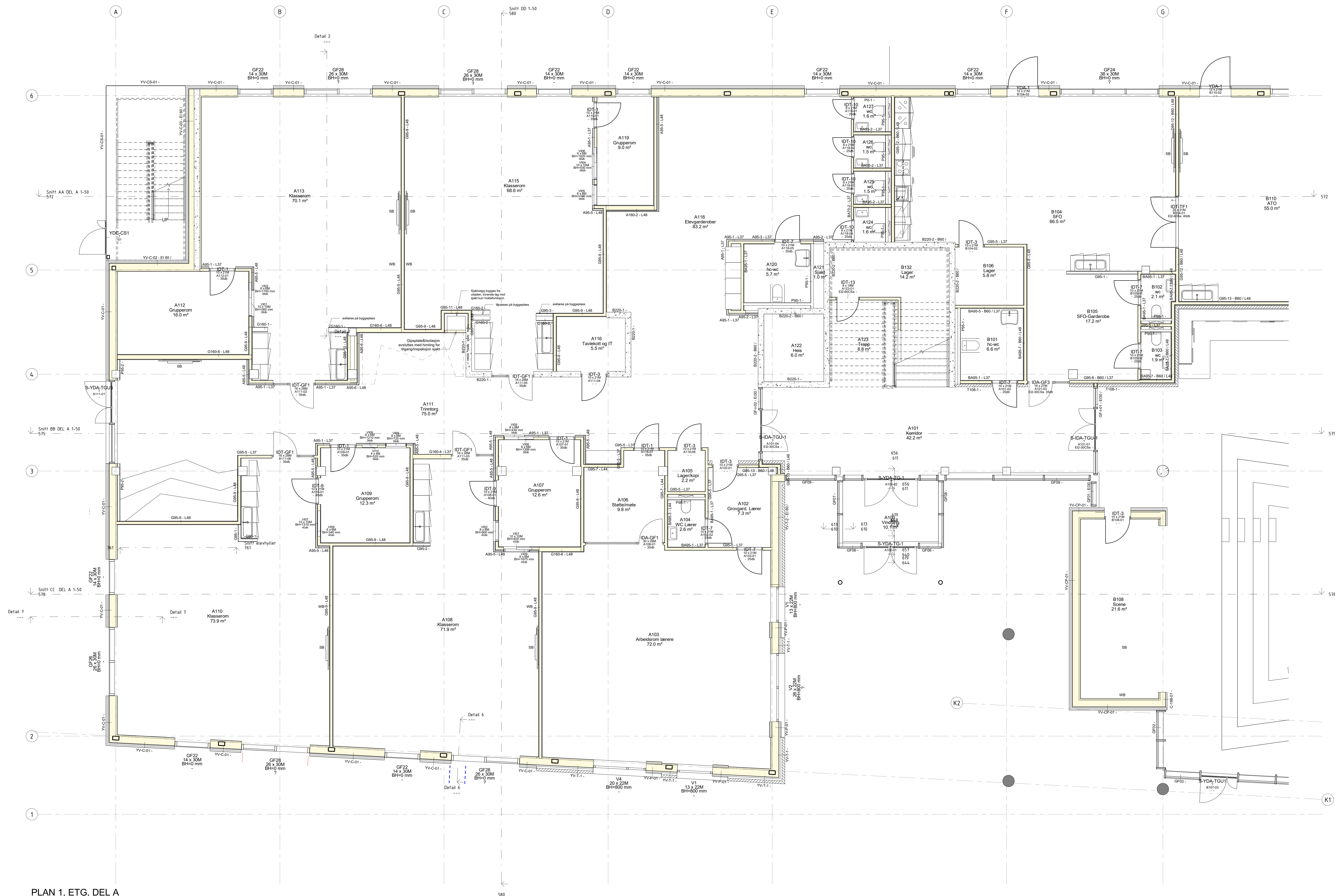
PLAN 1. ETG. DEL A 1:50
