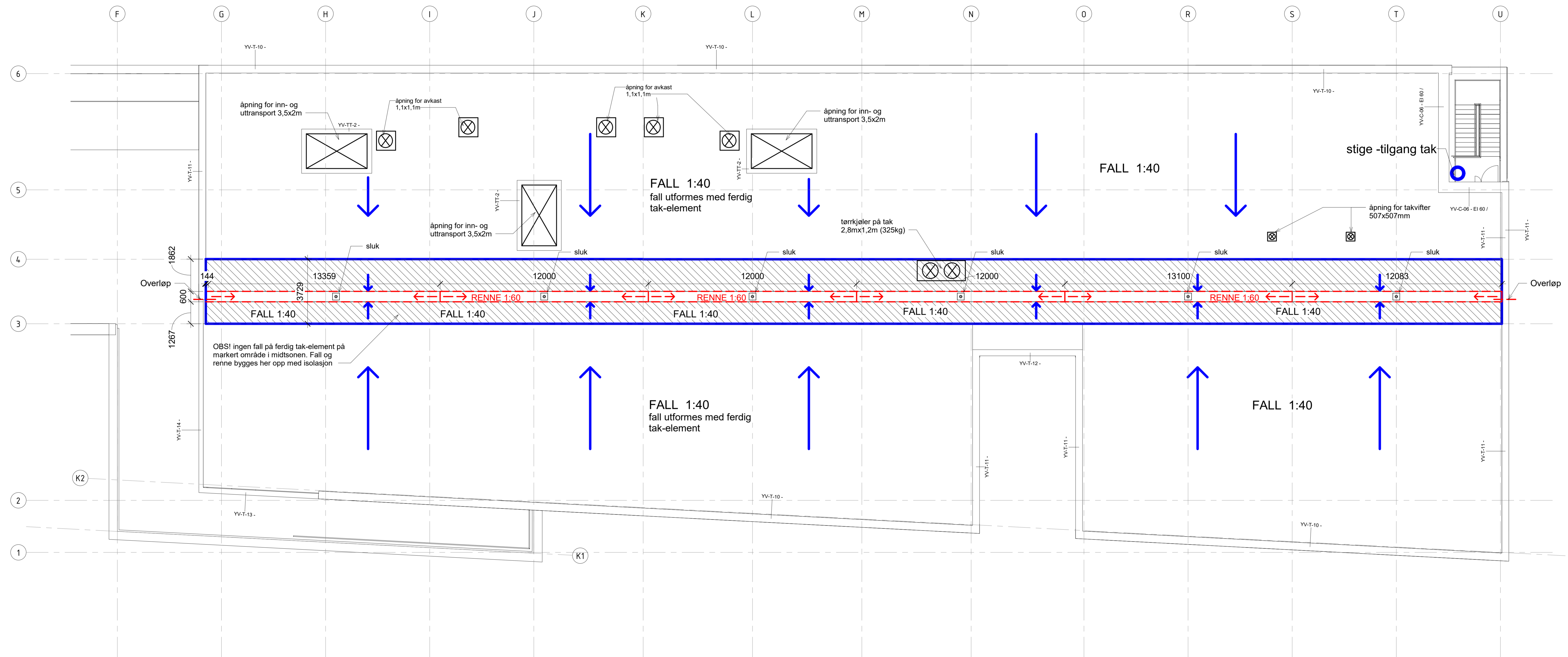
PLAN 5. ETG TAKPLAN 1:100
