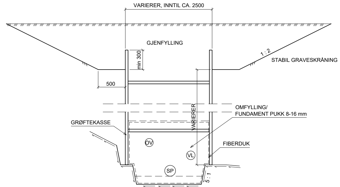
PRINSIPP GRØFTEKASSE
