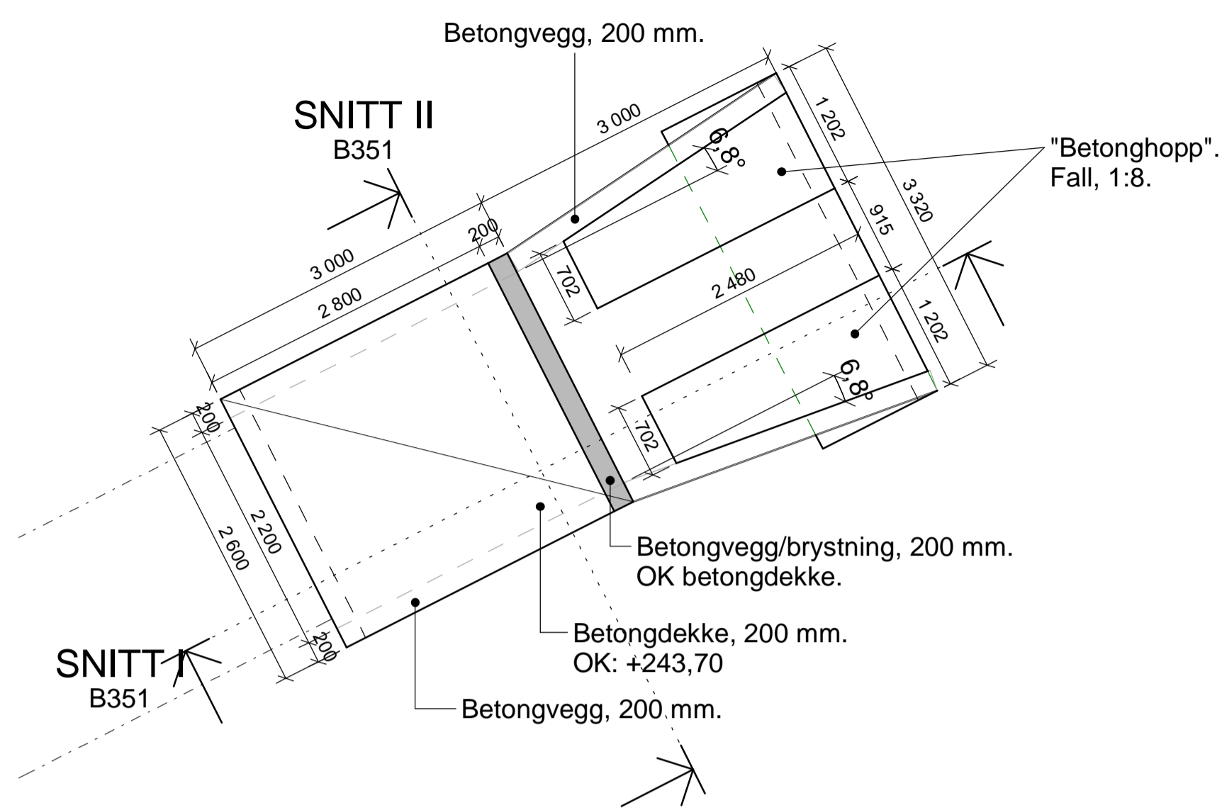
TOPP UTLØP 1 : 50
