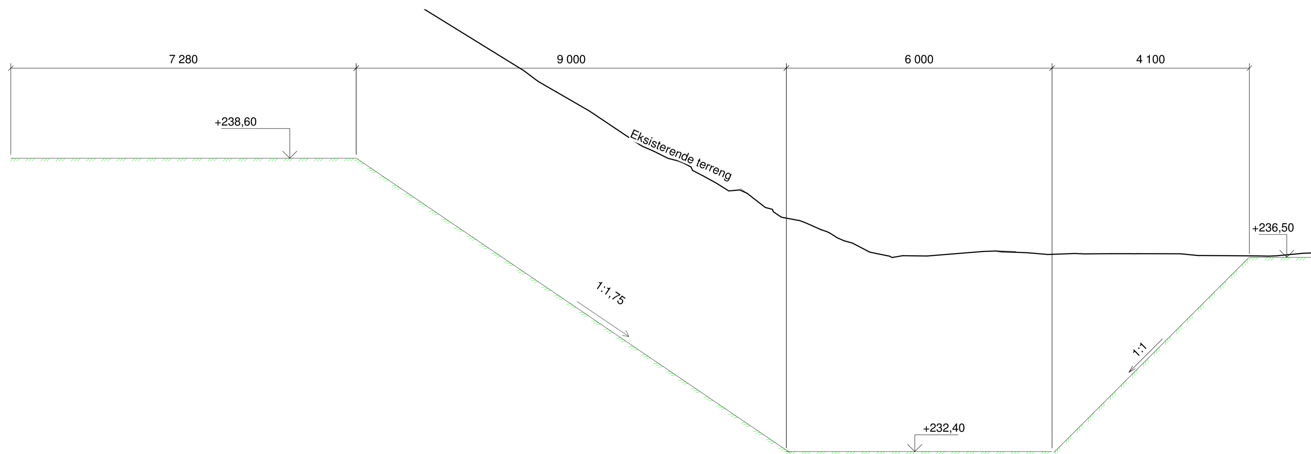
SNITT GRAVEPLAN UTLØP 1 : 50
