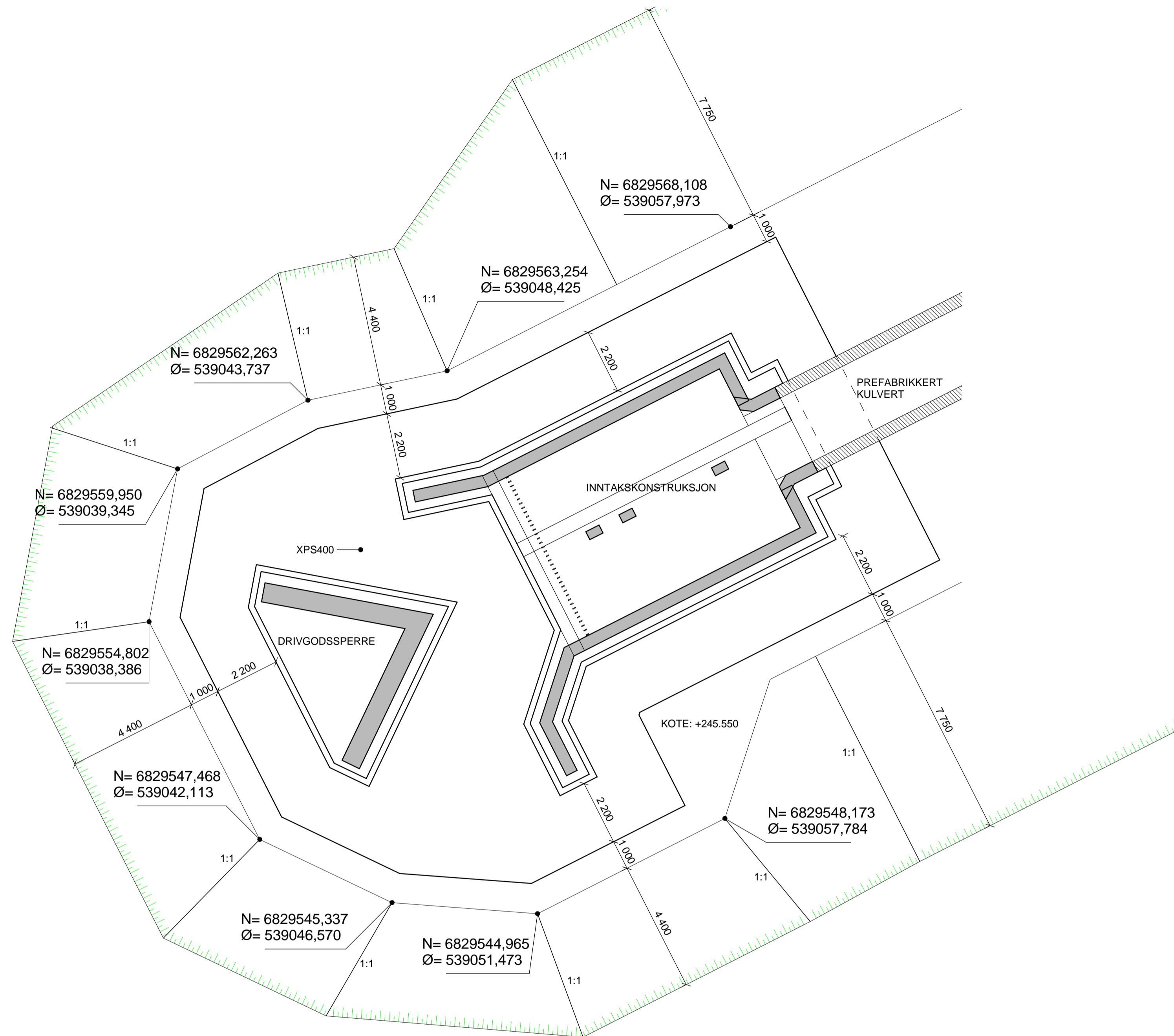
GRAVEPLAN INNSTAKSKONSTRUKSJON
