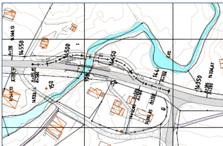
Tegning som viser interimsvegen
