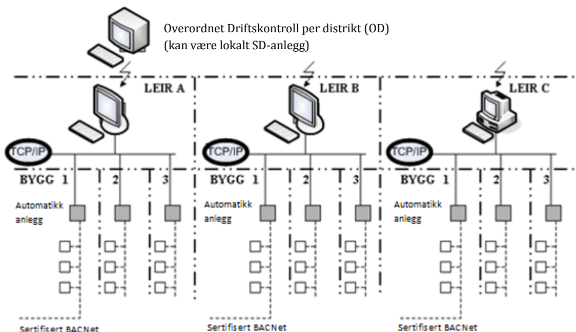
Figur 4. Prinsipiell nettløsning SD-anlegg og automatikkanlegg.
